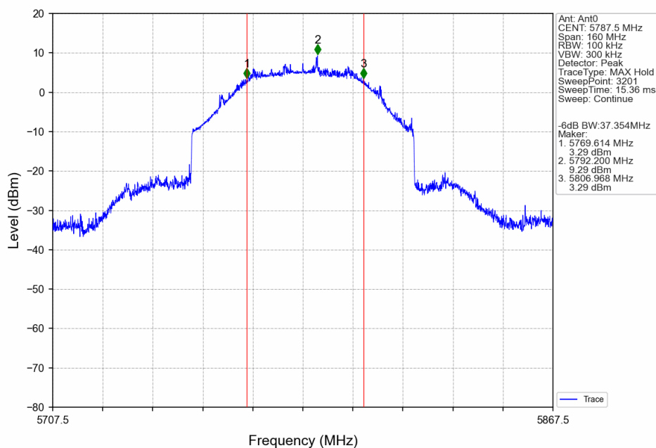
80M_MCH_5787.5MHz_Ant0_NTNV
