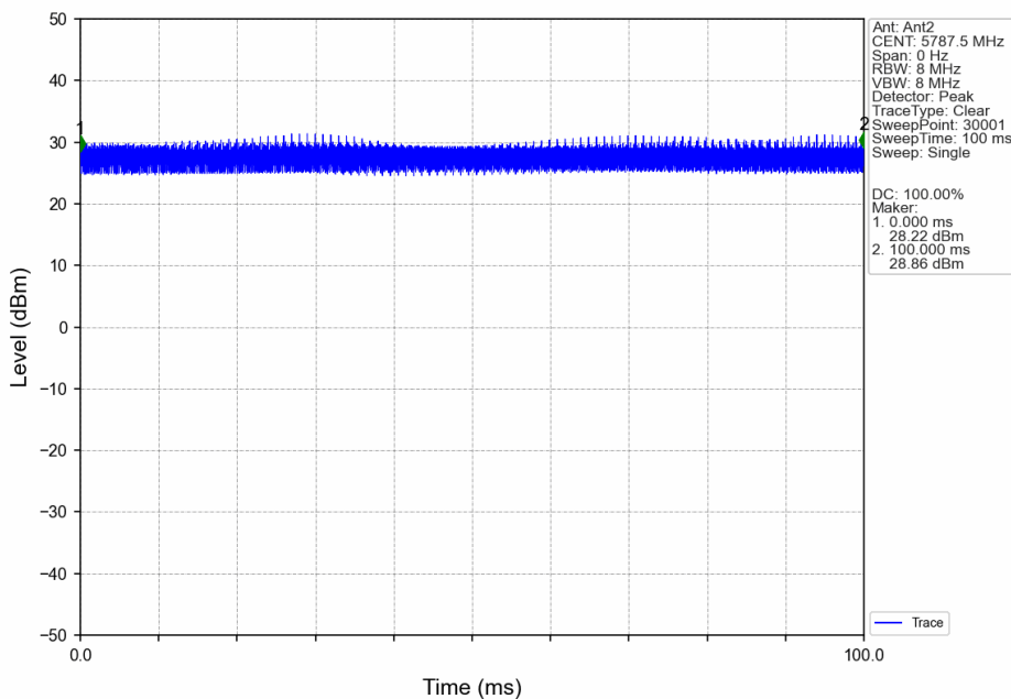
40M_MCH_5787.5MHz_Ant2_NTNV
