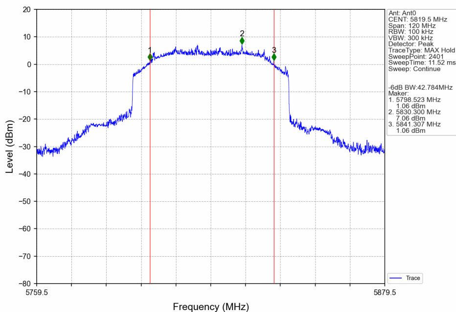
60M_HCH_5819.5MHz_Ant0_NTNV
