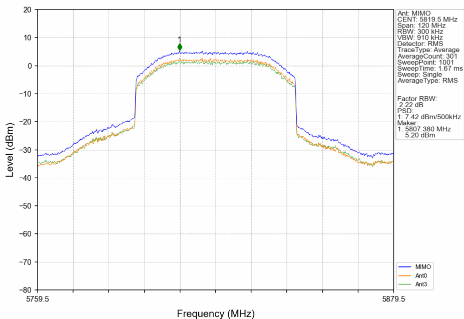
60M_HCH_5819.5MHz_MIMO_NTNV
