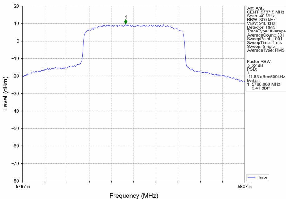
20M_MCH_5787.5MHz_Ant3_NTNV
