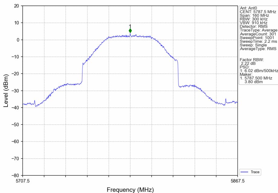
80M_MCH_5787.5MHz_Ant0_NTNV
