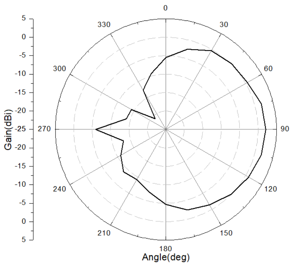
5.8G 俯仰面
