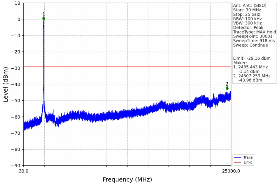
802.11n(HT40)_MCH_2437MHz_Ant1 (SISO)_NTNV
