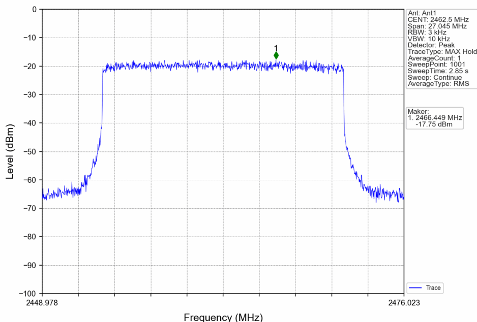
20M_HCH_2462.5MHz_MIMO_NTNV
