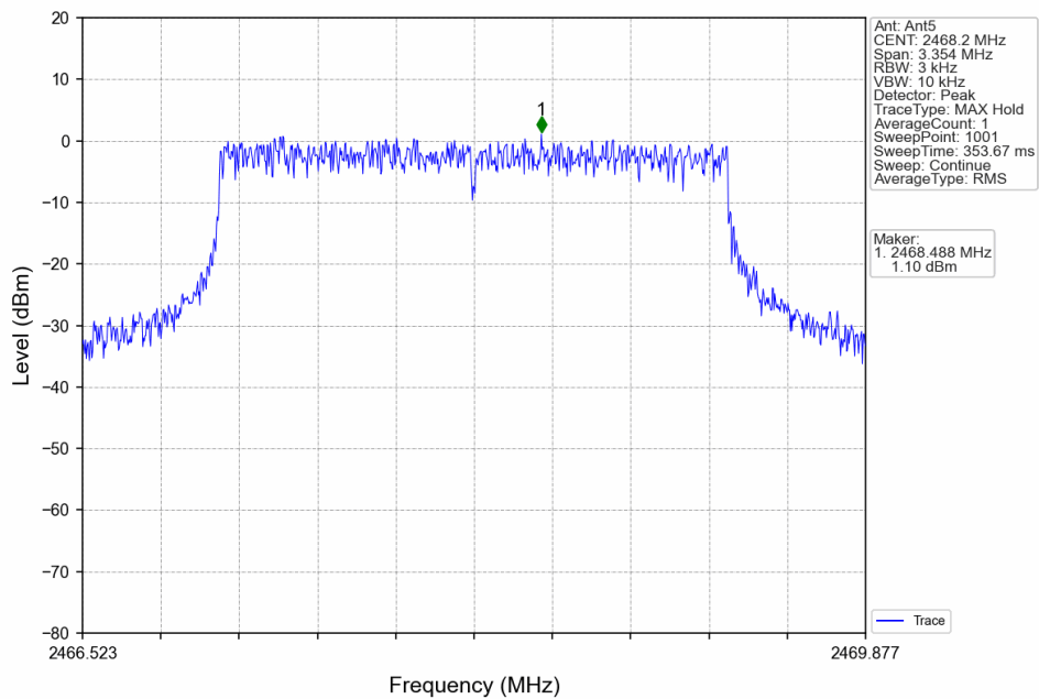
3M_HCH_2468.2MHz_Ant5_NTNV
