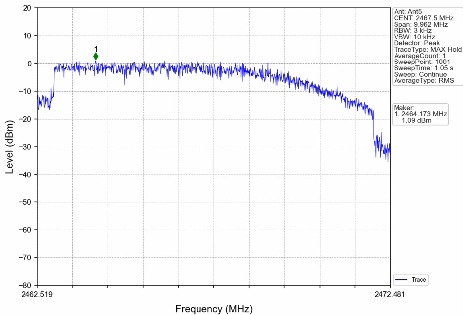
10M_HCH_2467.5MHz_Ant5_NTNV
