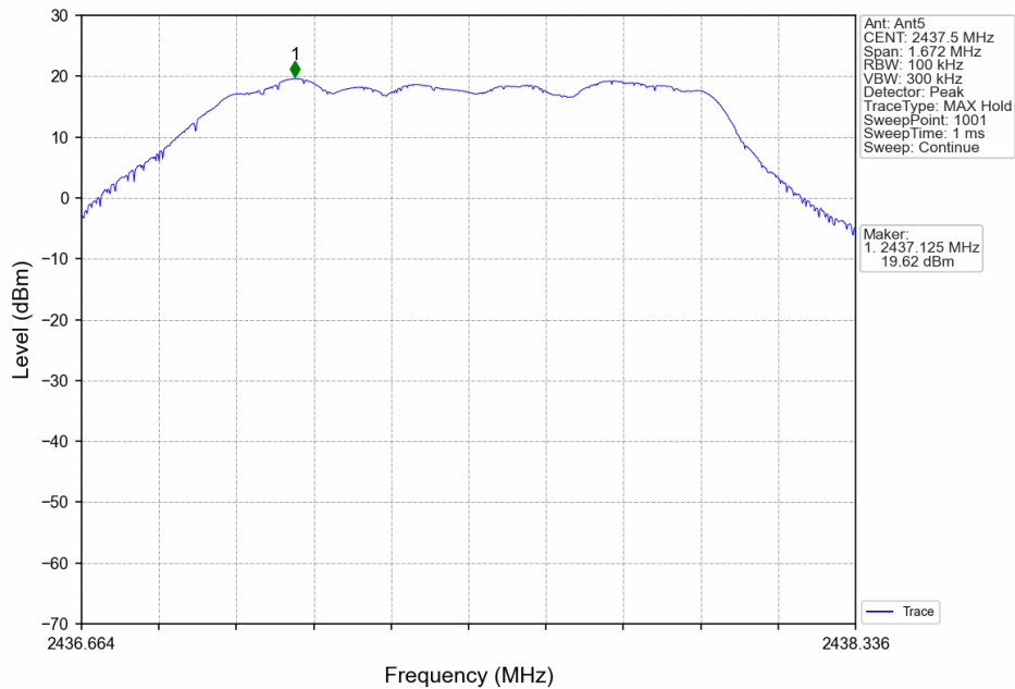
1.4M_MCH_2437.5MHz_Ant5_NTNV
