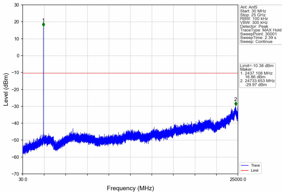
1.4M_MCH_2437.5MHz_Ant5_NTNV
