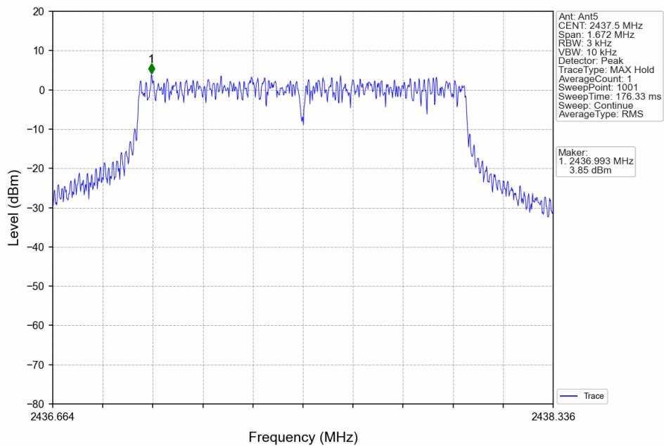
1.4M_MCH_2437.5MHz_Ant5_NTNV
