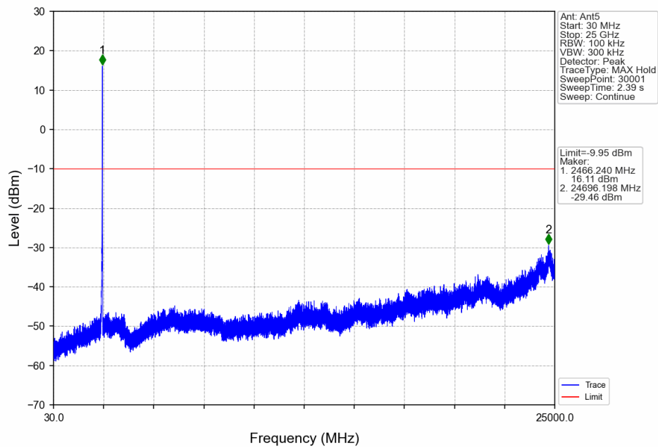
10M_HCH_2467.5MHz_Ant5_NTNV
