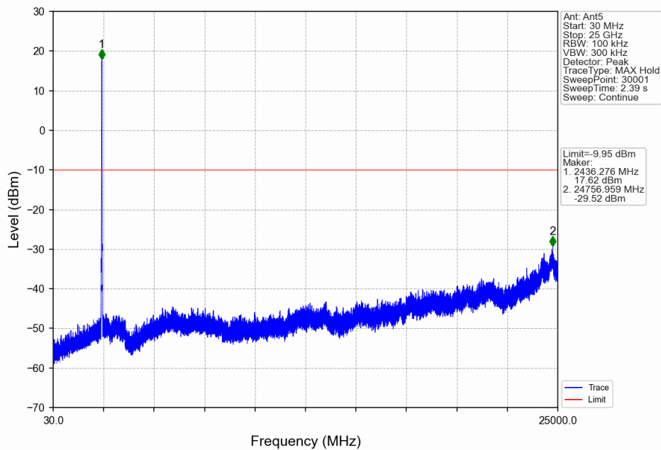
10M_MCH_2437.5MHz_Ant5_NTNV
