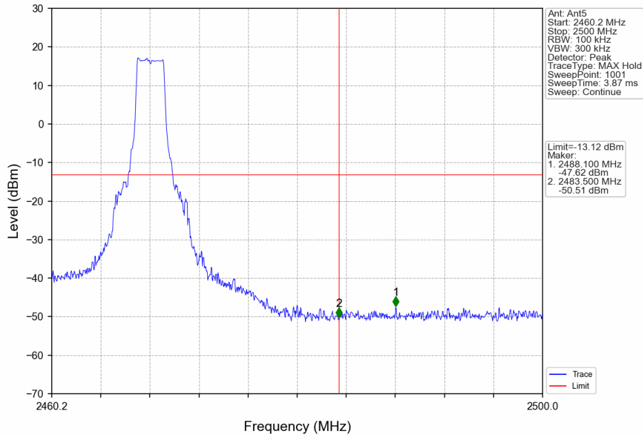
3M_HCH_2468.2MHz_Ant5_NTNV
