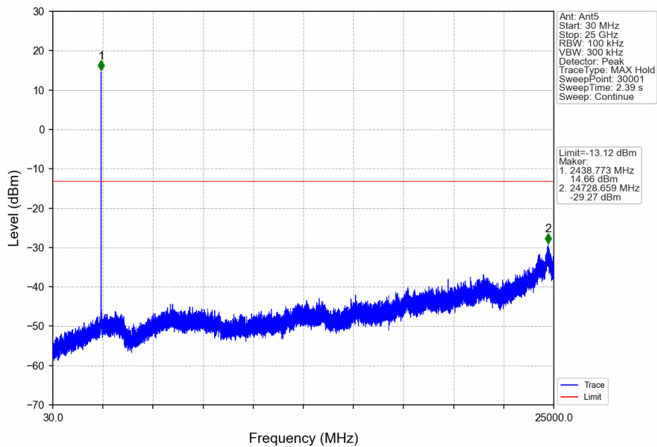
3M_MCH_2438.5MHz_Ant5_NTNV
