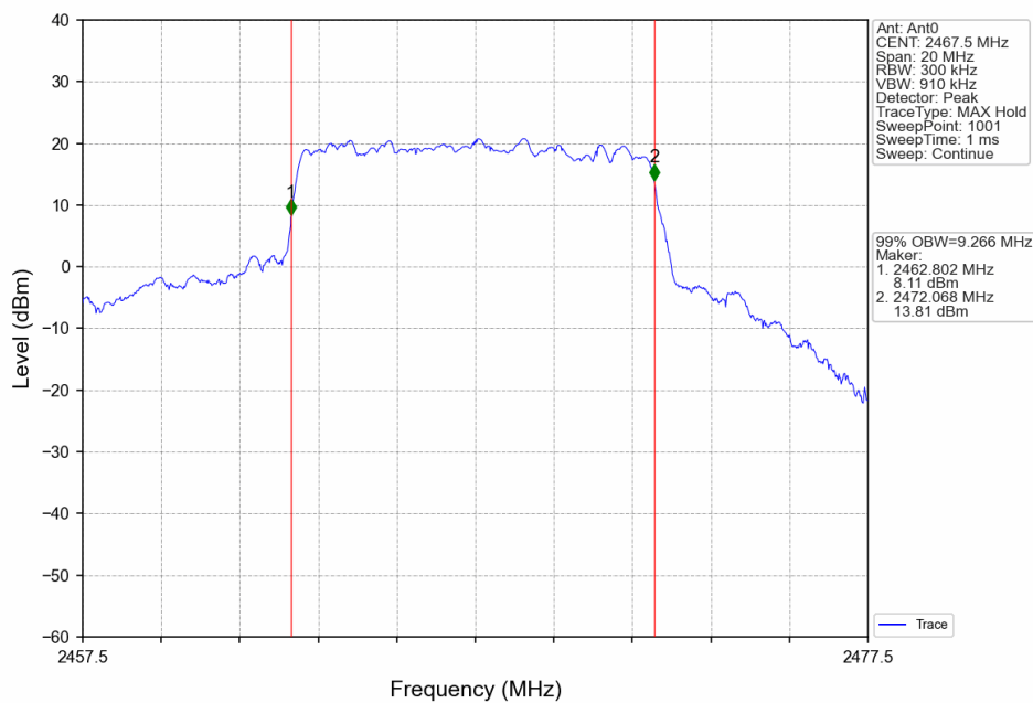
10M_HCH_2467.5MHz_Ant0_NTNV
