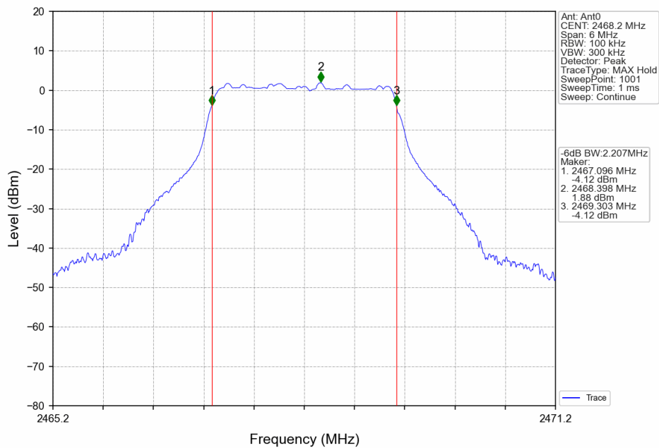
3M_HCH_2468.2MHz_Ant0_NTNV
