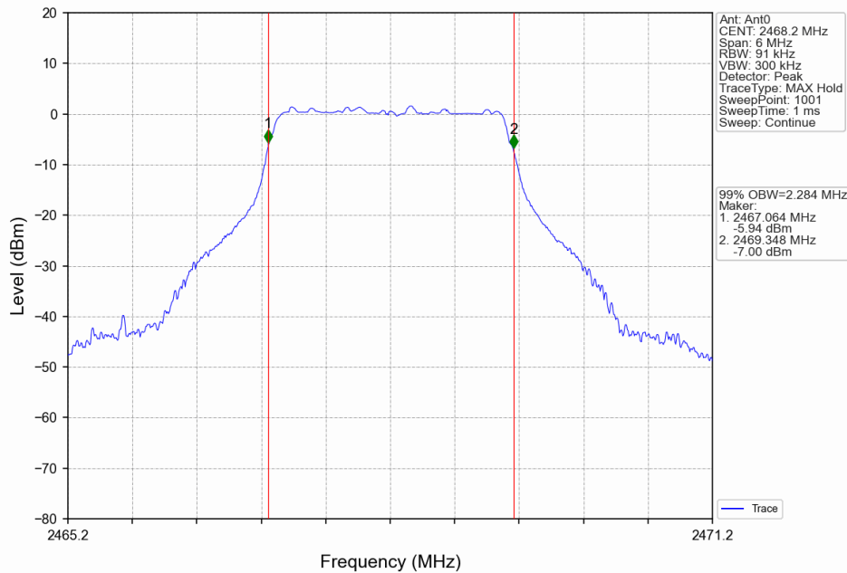
3M_HCH_2468.2MHz_Ant0_NTNV
