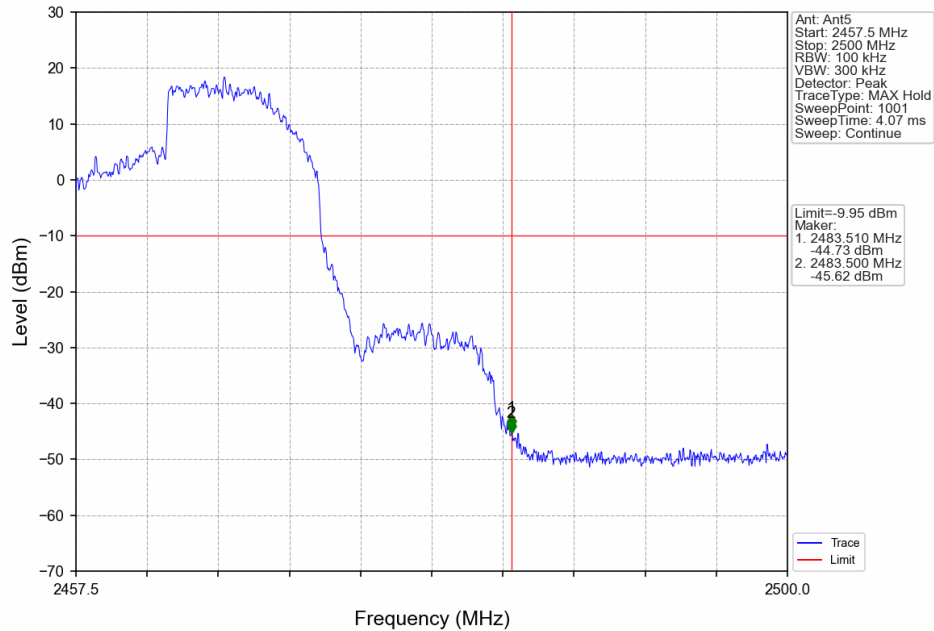
10M_HCH_2467.5MHz_Ant5_NTNV
