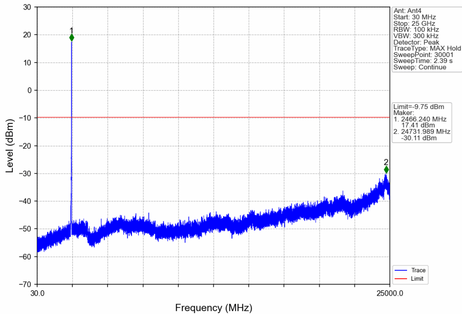
10M_HCH_2467.5MHz_Ant4_NTNV
