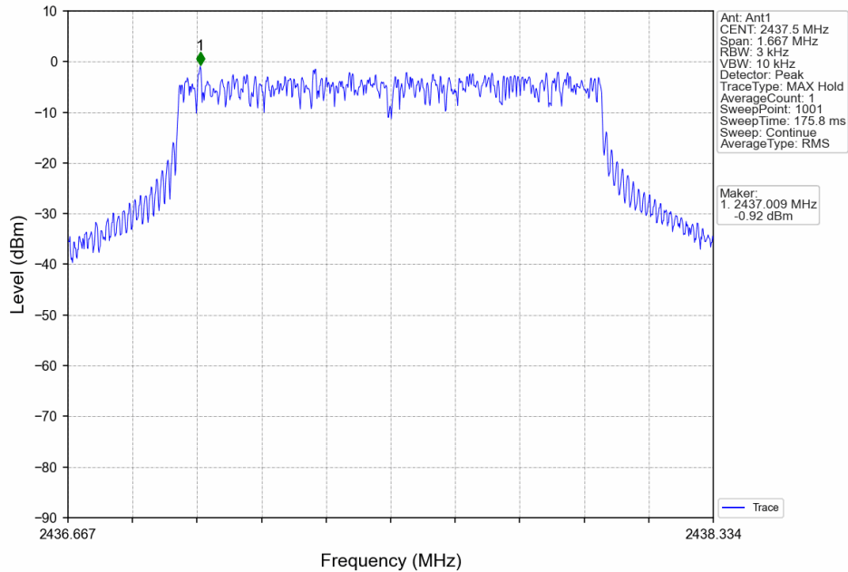
1.4M_MCH_2437.5MHz_MIMO_NTNV
