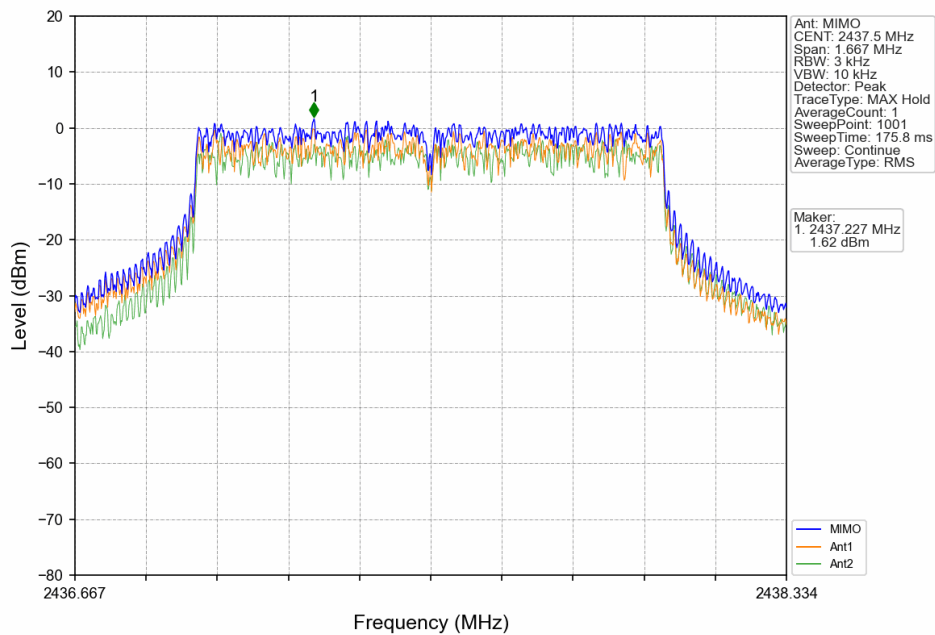
1.4M_MCH_2437.5MHz_MIMO_NTNV
