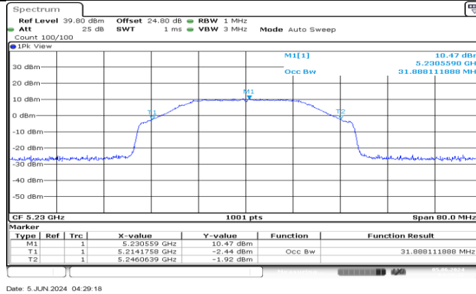
SRD 40MHz_Ant0_5230
