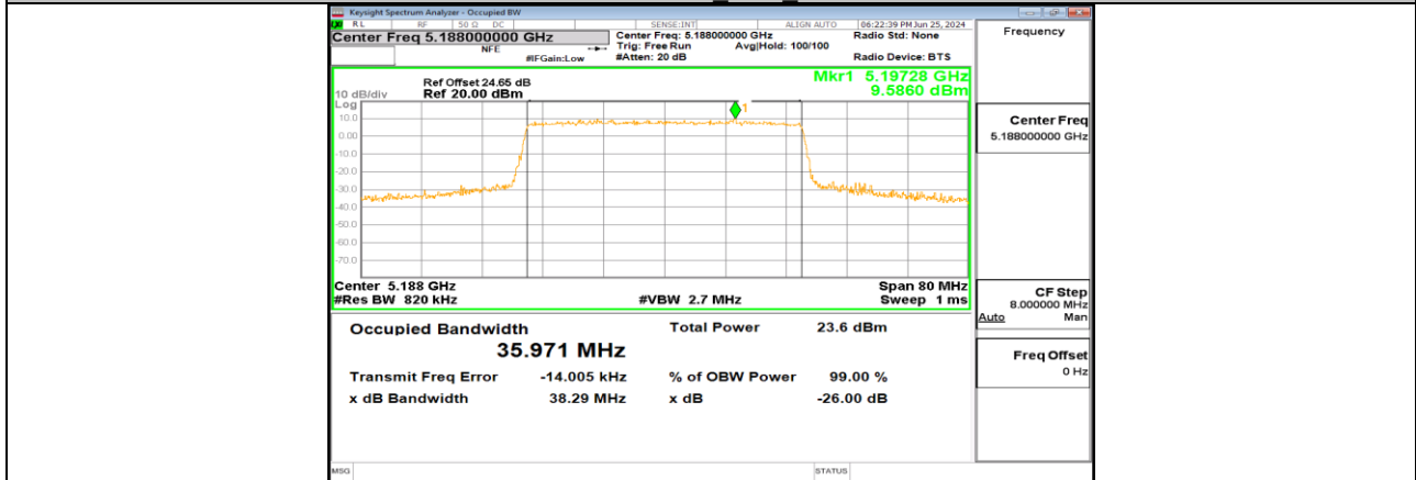
SRD 40MHz_Ant0_5188
