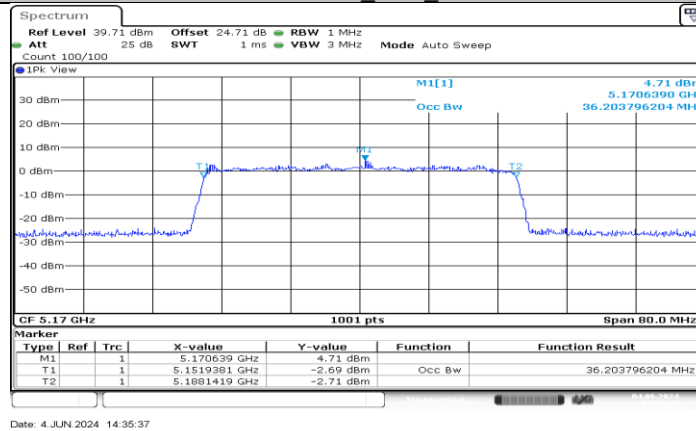
SRD 40MHz_Ant1_5170
