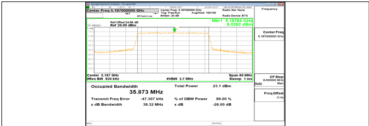
SRD 40MHz_Ant0_5187
