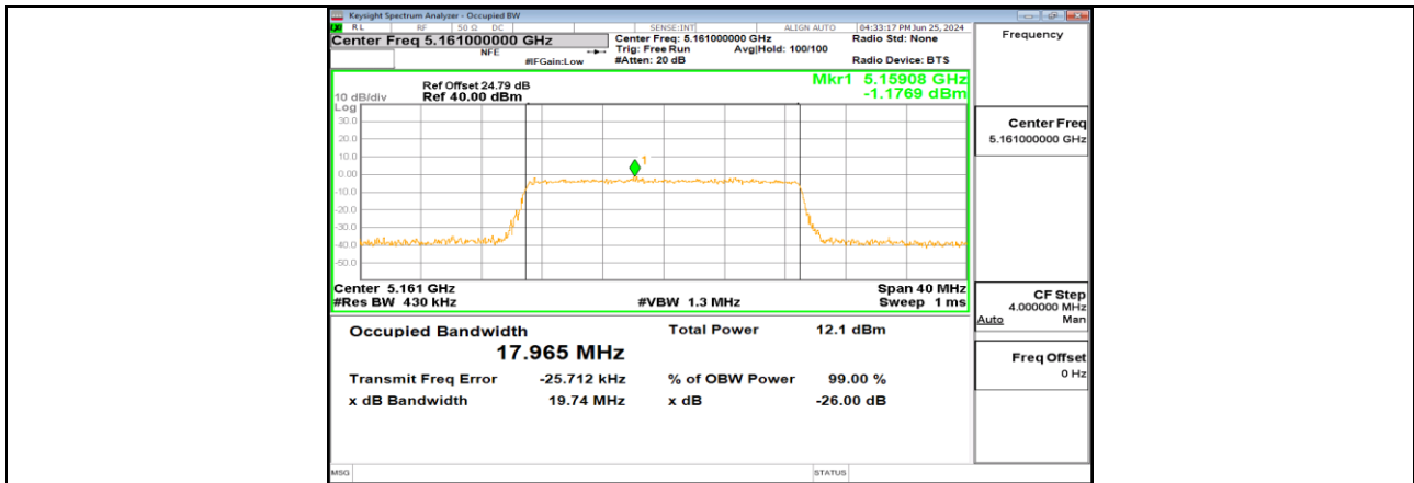
SRD 20MHz_Ant1_5161
