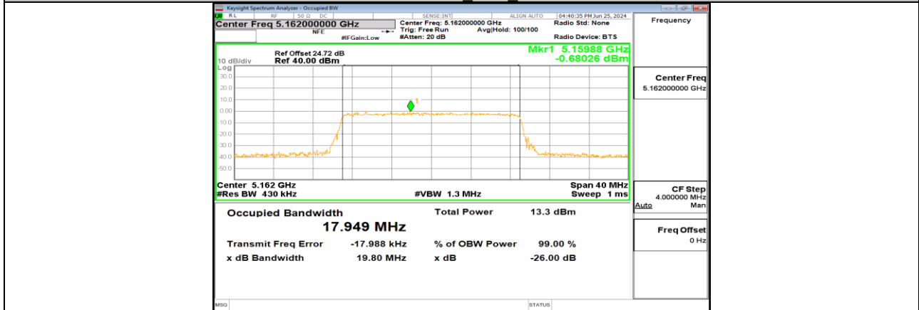
SRD 20MHz_Ant0_5162
