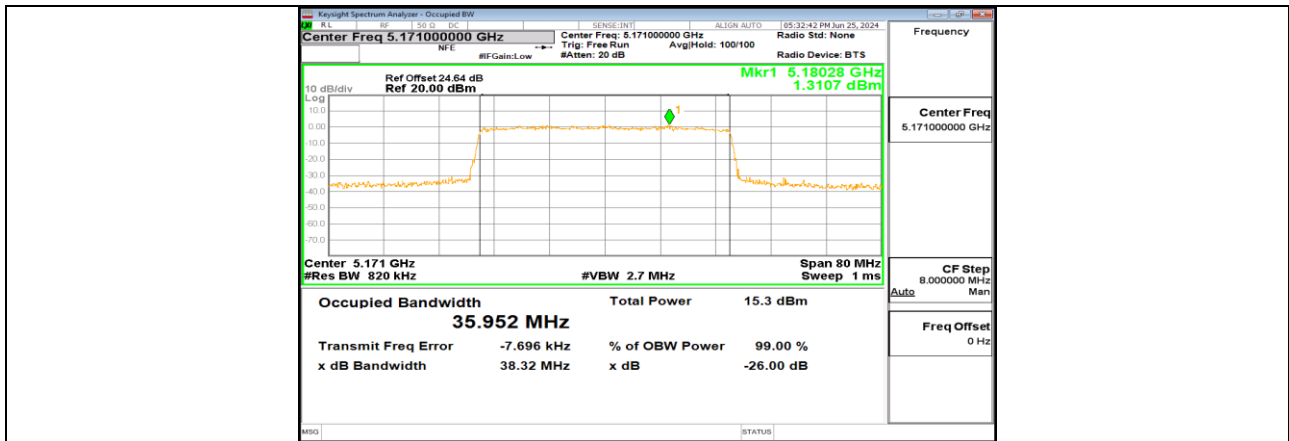
SRD 40MHz_Ant0_5171
