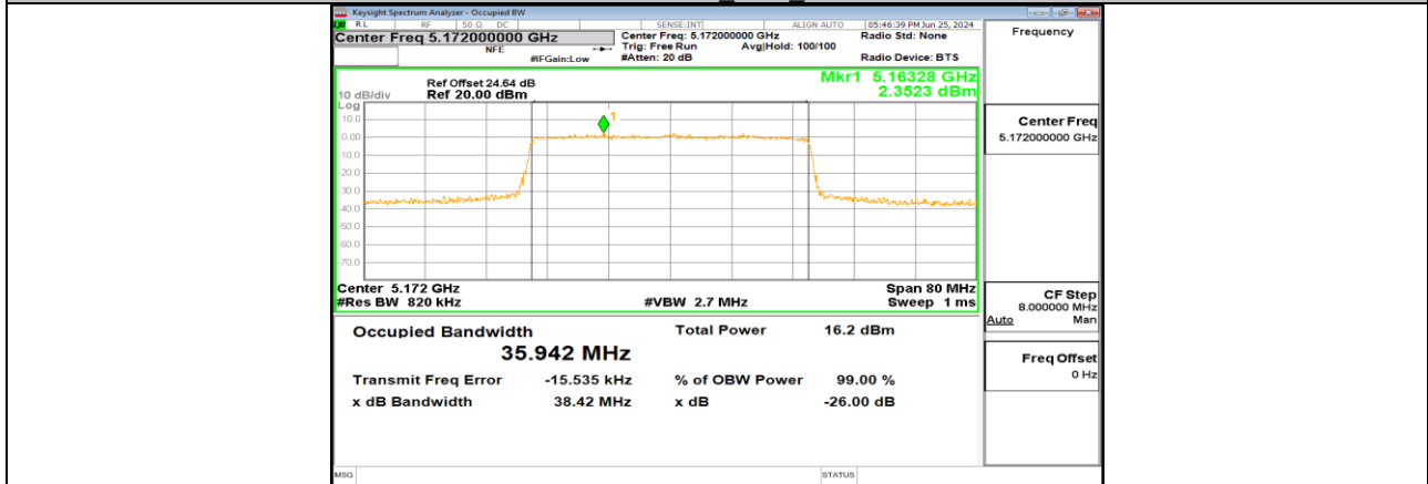
SRD 40MHz_Ant0_5172
