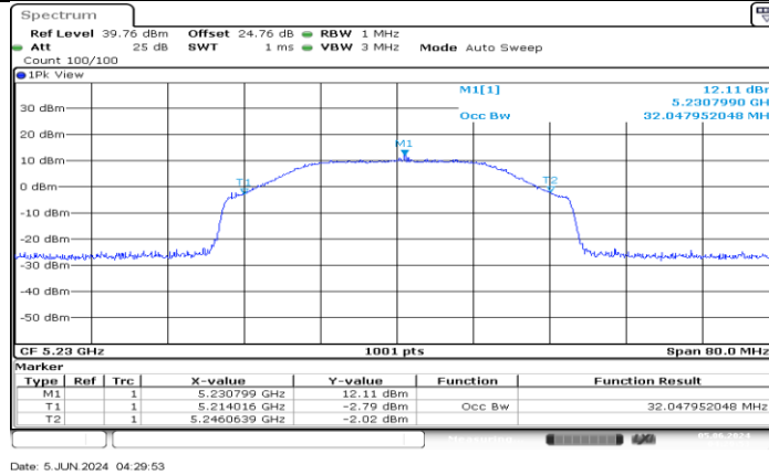
SRD 40MHz_Ant1_5230
