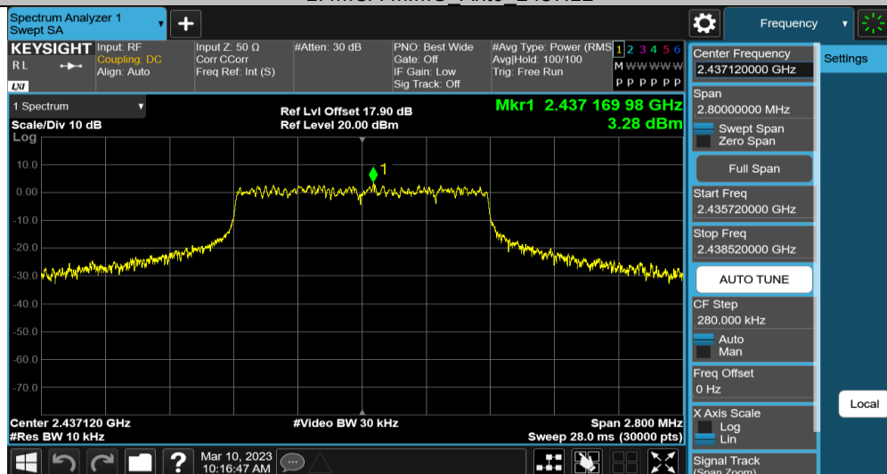
1.4MCA-MIMO Ant0 2437.12
