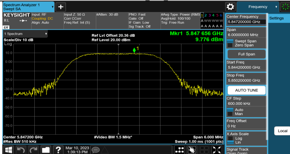
3MCA-MIMO_Ant3_5847.2
