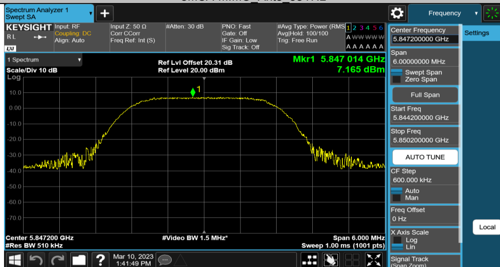
3MCA-MIMO_Ant3_5847.2
