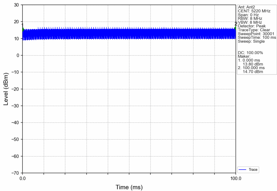
60M_HCH_5220MHz_Ant2_NTNV
