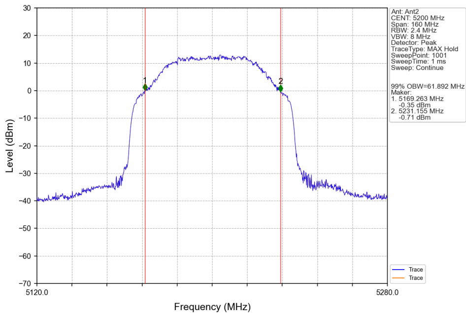
80M_MCH_5200MHz_Ant2_NTNV
