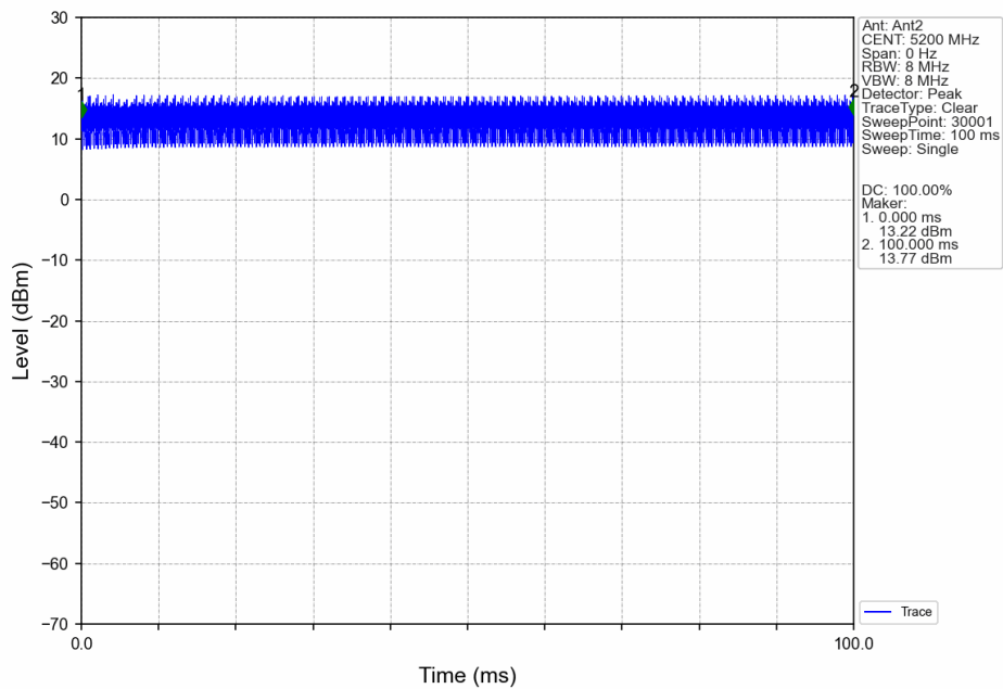
80M_MCH_5200MHz_Ant2_NTNV
