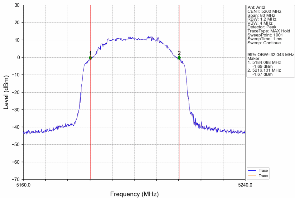
40M_MCH_5200MHz_Ant2_NTNV
