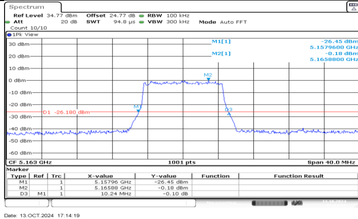
SRD 10M_Ant0_5163
