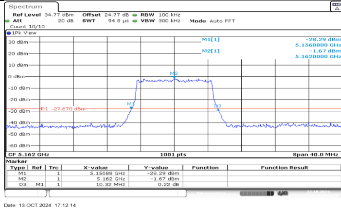
SRD 10M_Ant0_5162
