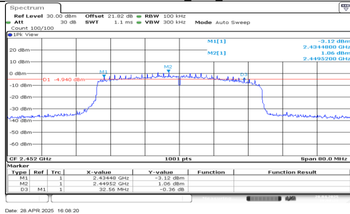
11AX40MIMO_Ant3_2452
