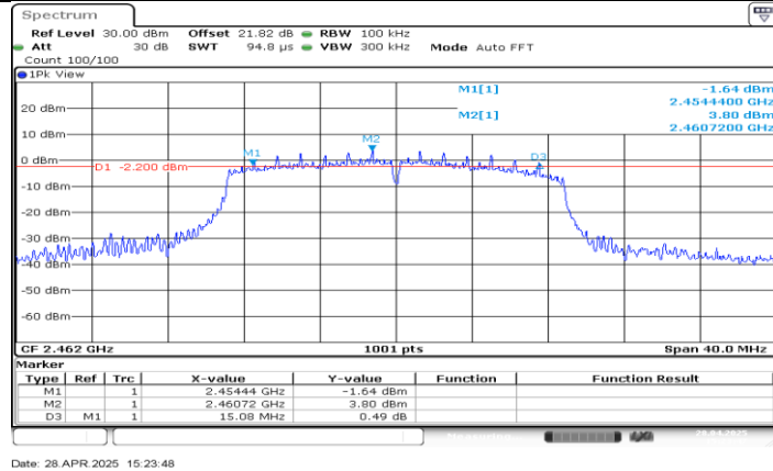
11N20MIMO_Ant3_2462
