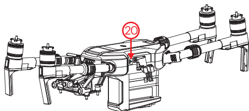
折叠状态
