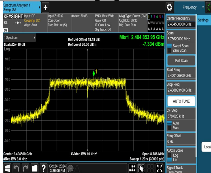
5MHz_Ant2_2404.5
