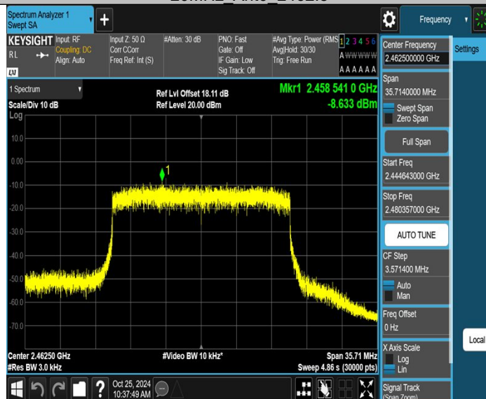
20MHz Ant2 2462.5
