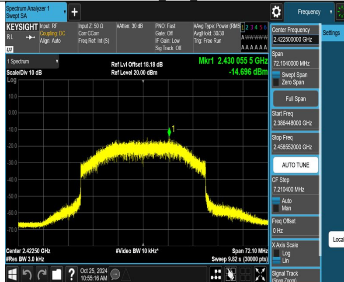
40MHz_Ant2_2422.5
