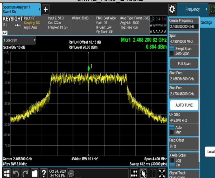
3MHz_Ant2_2468.2
