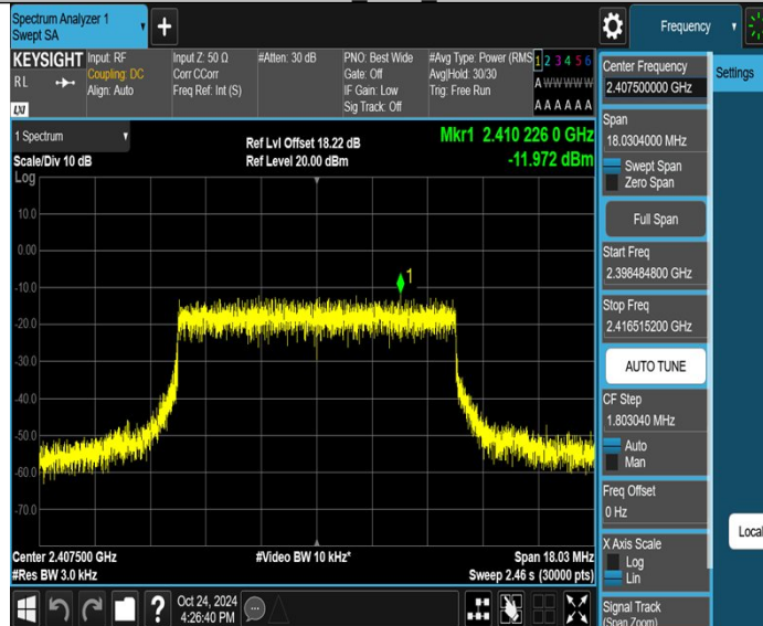
10MHz_Ant2_2407.5
