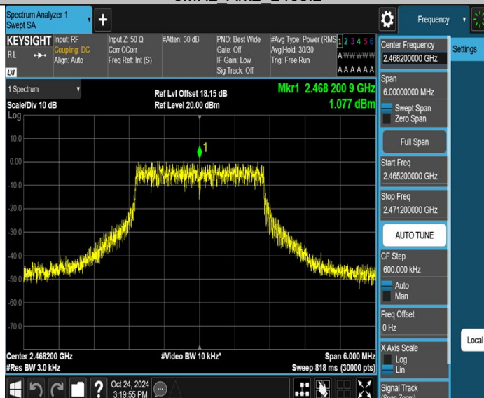
3MHz_Ant2_2468.2
