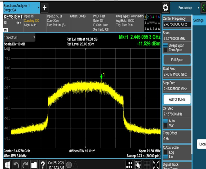
40MHz_Ant0_2437.5
