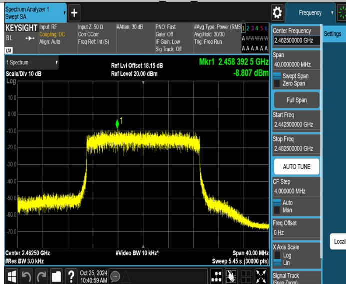
20MHz Ant2 2462.5
