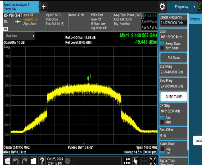
60MHz Ant0 2437.5
