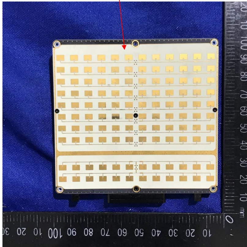
Antenna
