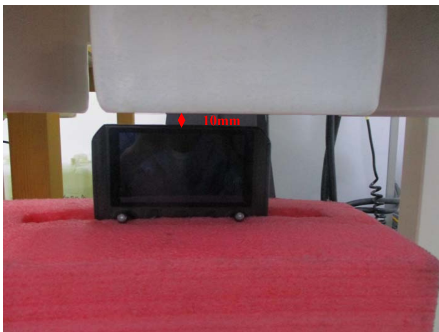
Test Position_Bottom(Wi-Fi) (10mm)
