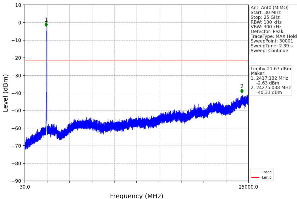
802.11n(HT40)_LCH_2422MHz_Ant0 (MIMO)_NTNV
