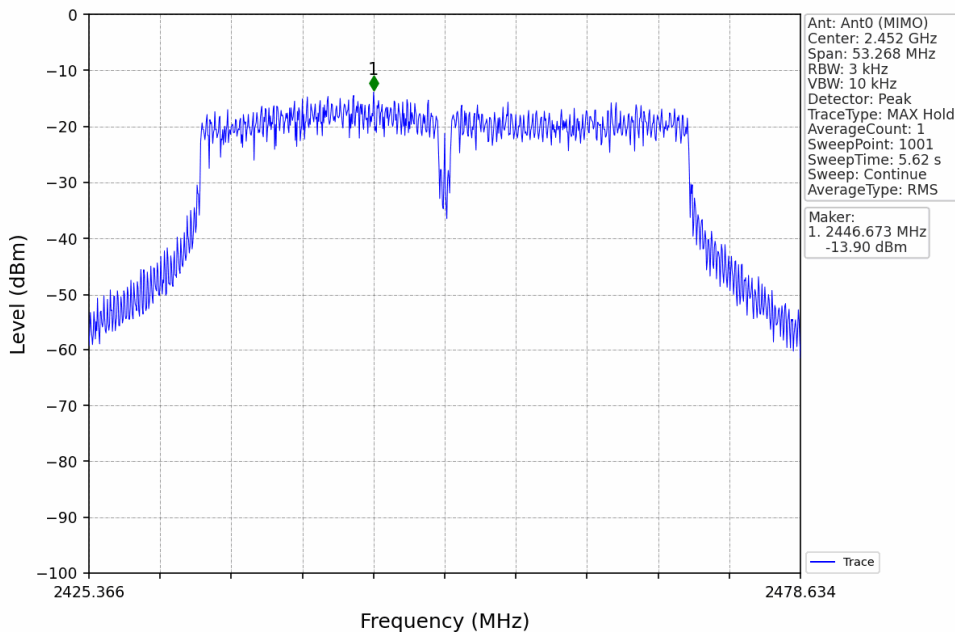
802.11n(HT40)_HCH_2452MHz_Ant0 (MIMO)_NTNV
