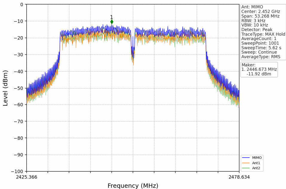
802.11n(HT40)_HCH_2452MHz_MIMO_NTNV
