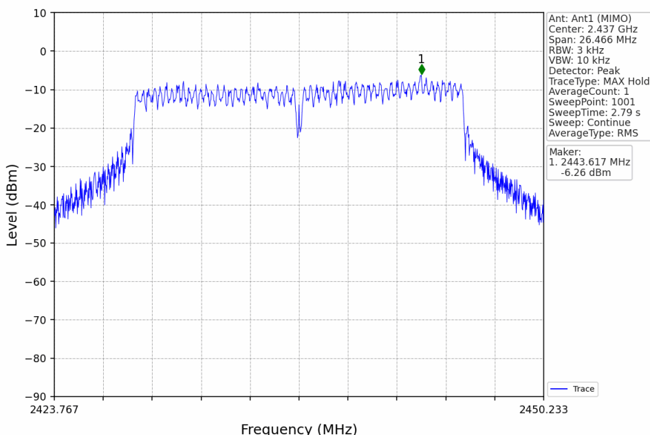
802.11n(HT20)_MCH_2437MHz_MIMO_NTNV
