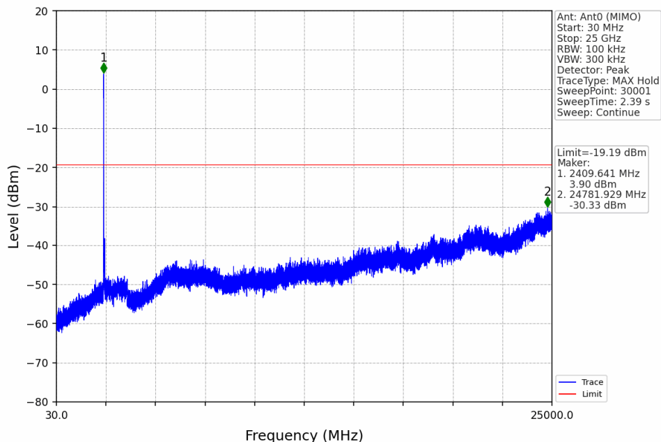
802.11n(HT20)_LCH_2412MHz_Ant0 (MIMO)_NTNV
