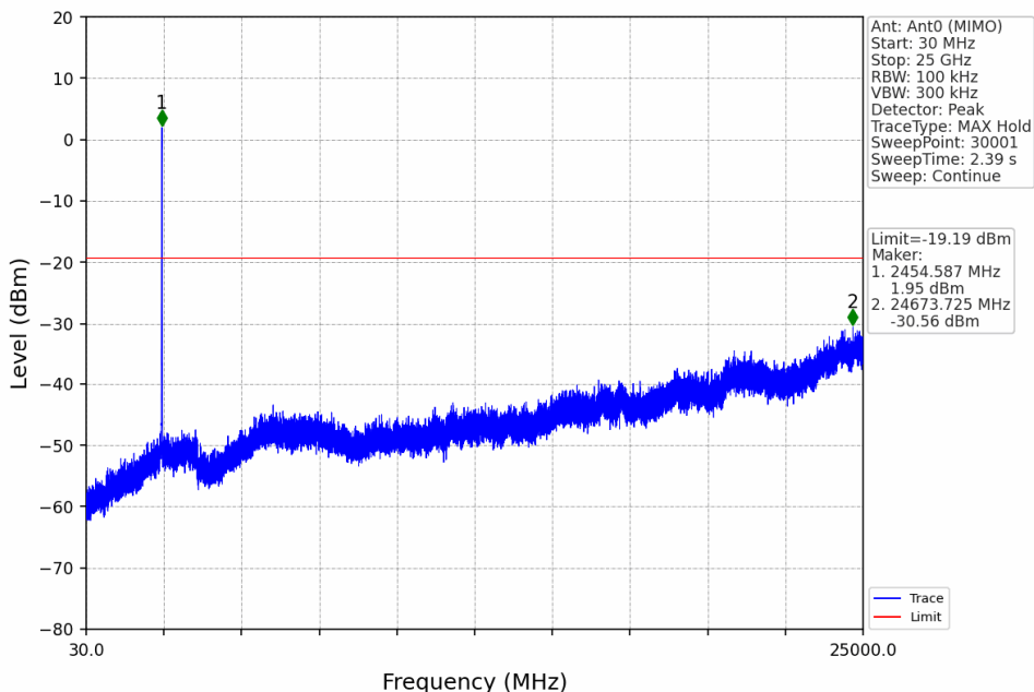
802.11n(HT20)_HCH_2462MHz_Ant0 (MIMO)_NTNV
