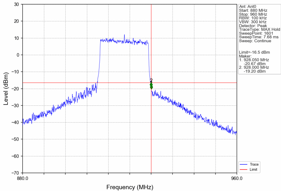
20M_HCH_918MHz_Ant0_NTNV
