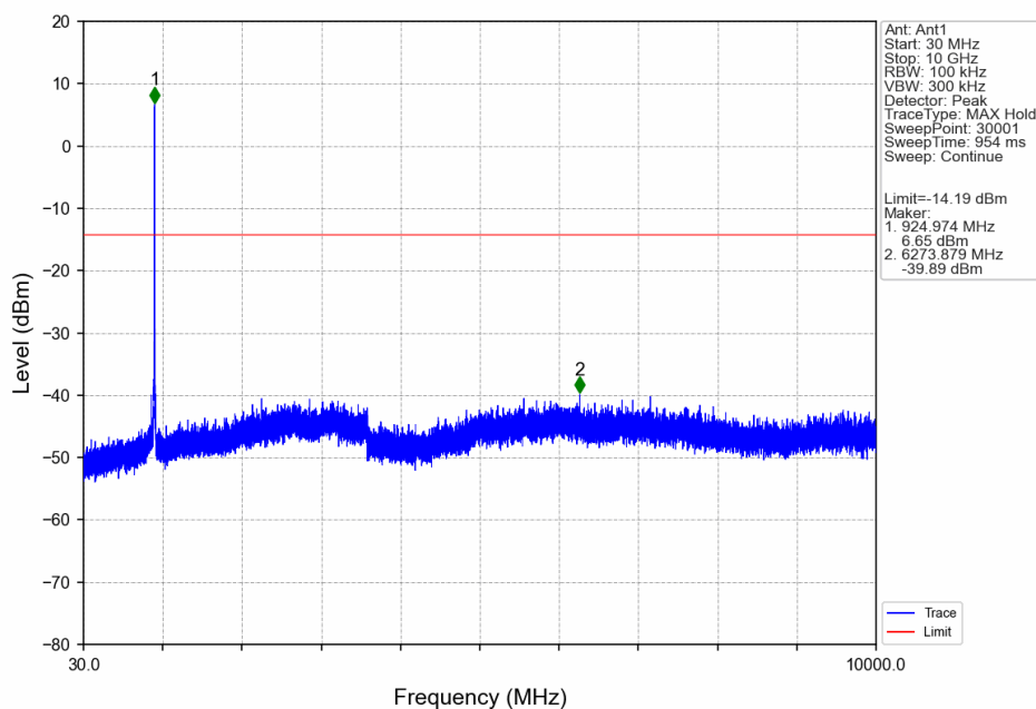
10M_HCH_923MHz_Ant1_NTNV
