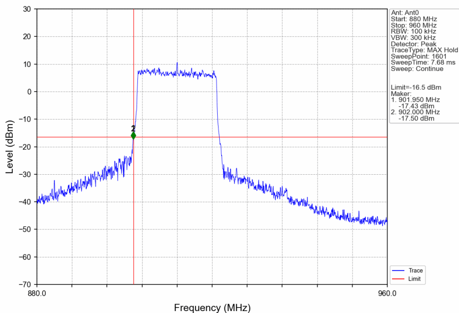
20M_LCH_912MHz_Ant0_NTNV
