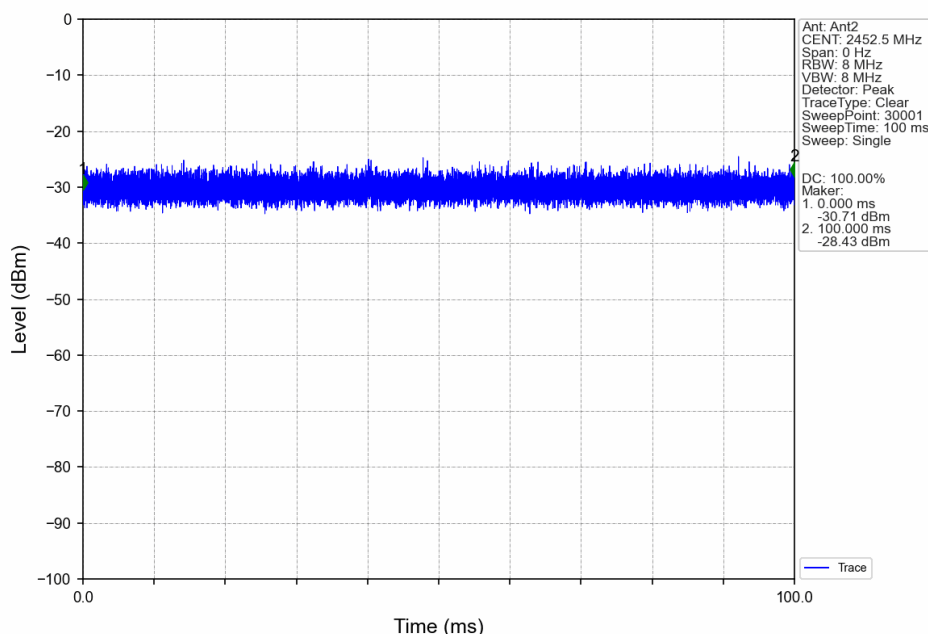
40M_HCH_2452.5MHz_Ant2_NTNV
