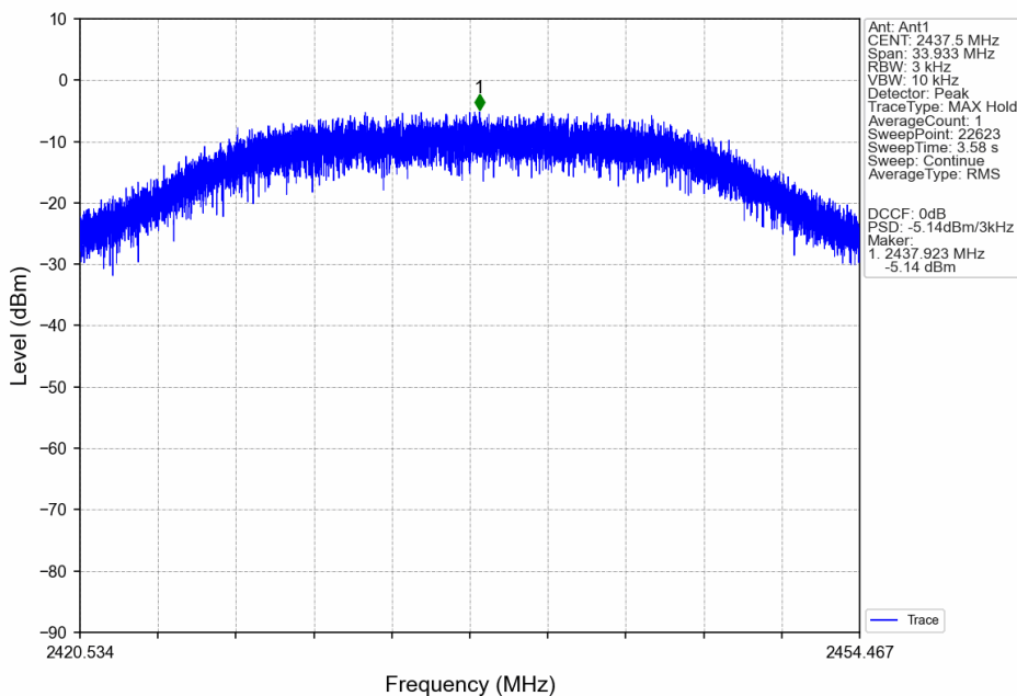
40M_MCH_2437.5MHz_Ant1_NTNV
