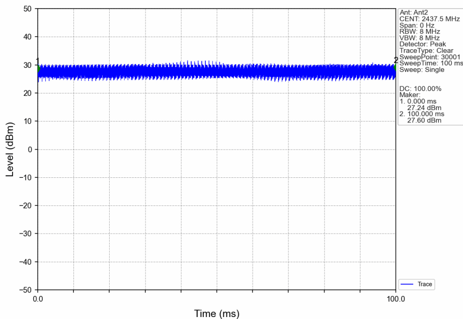
20M_MCH_2437.5MHz_Ant2_NTNV
