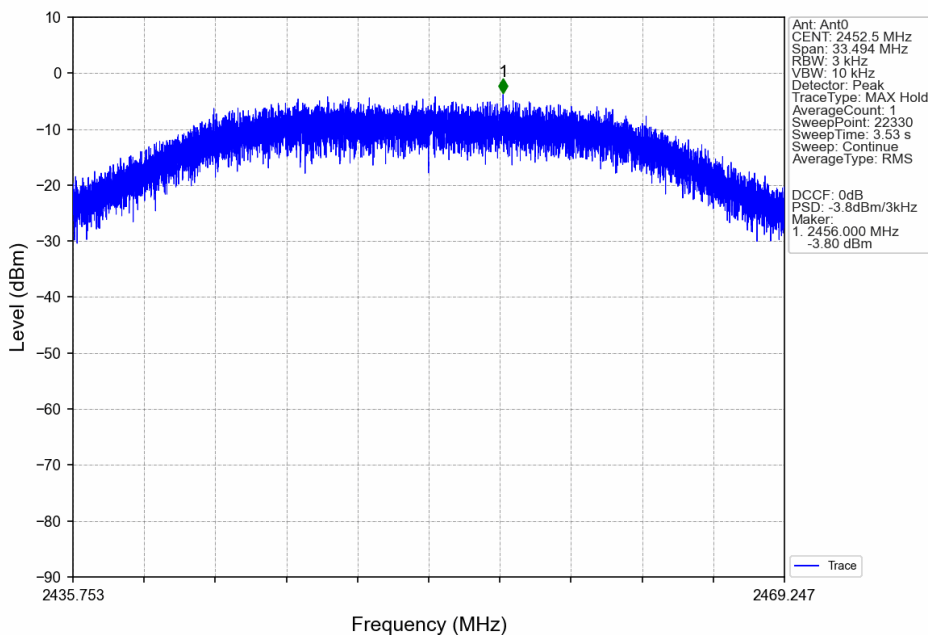
40M_HCH_2452.5MHz_Ant0_NTNV
