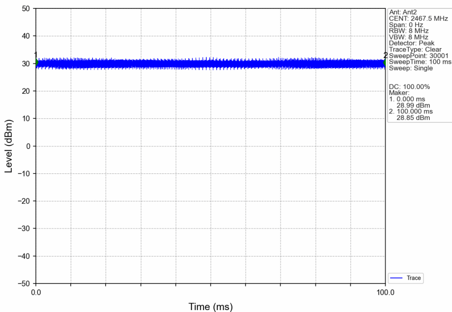
10M_HCH_2467.5MHz_Ant2_NTNV
