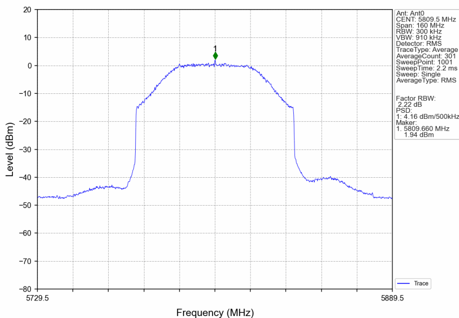
80M_HCH_5809.5MHz_Ant0_NTNV
