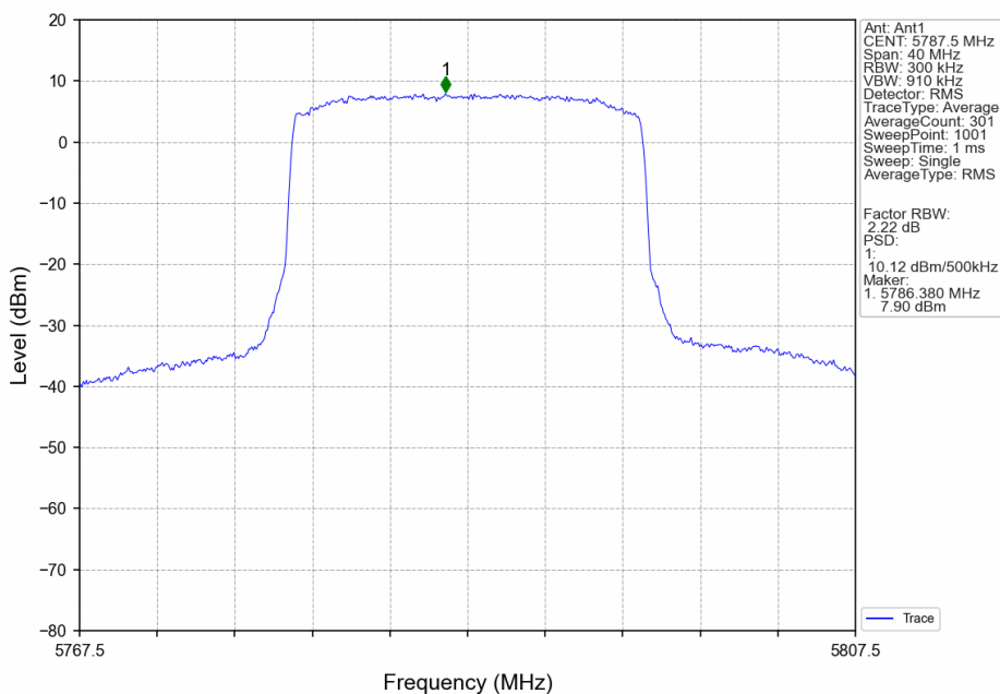
20M_MCH_5787.5MHz_MIMO_NTNV
