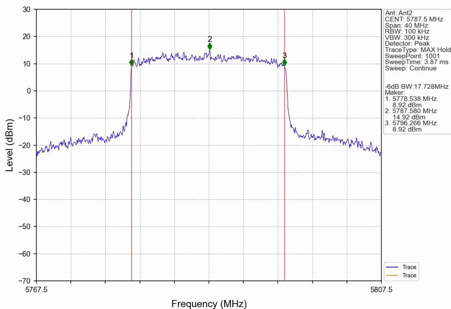
20M_MCH_5787.5MHz_Ant2_NTNV
