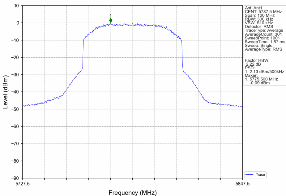
60M_MCH_5787.5MHz_MIMO_NTNV
