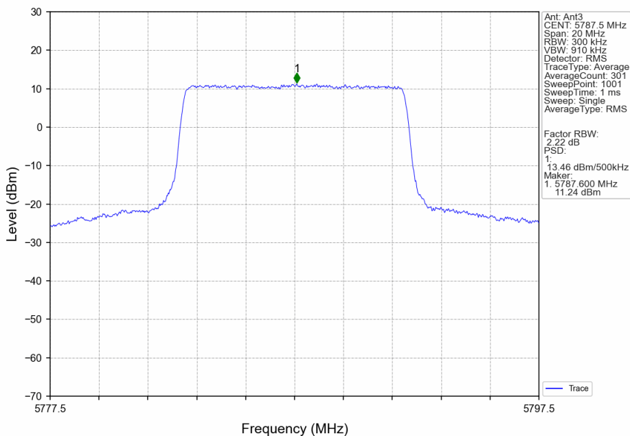
10M_MCH_5787.5MHz_Ant3_NTNV
