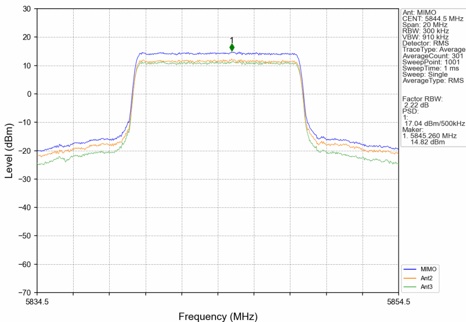
10M_HCH_5844.5MHz_MIMO_NTNV
