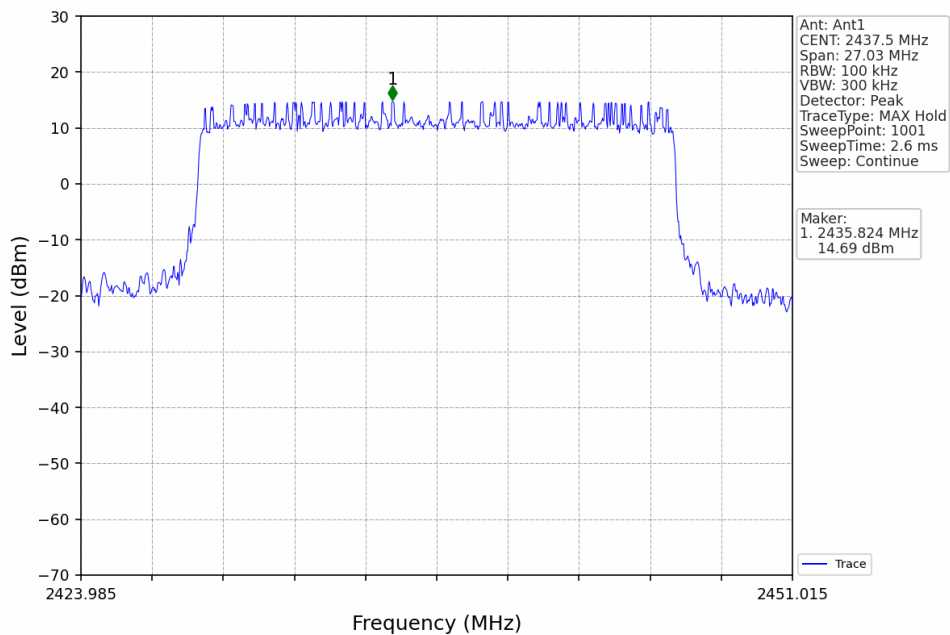
20M_MCH_2437.5MHz_Ant1_NTNV
