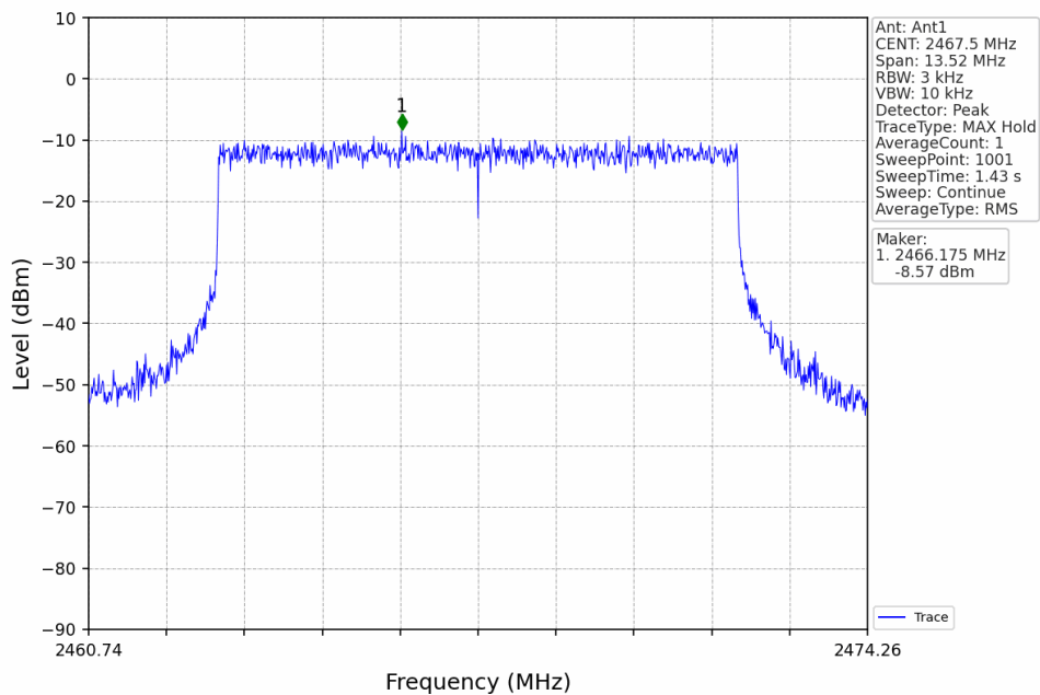
10M_HCH_2467.5MHz_Ant1_NTNV
