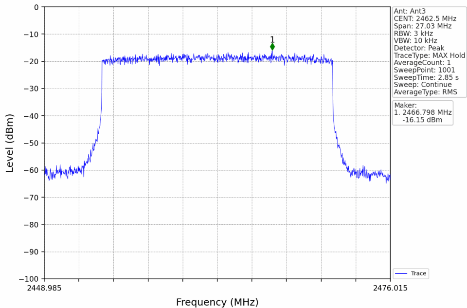
20M_HCH_2462.5MHz_Ant3_NTNV
