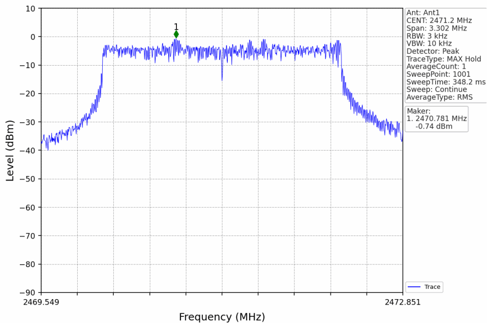
3M_HCH_2471.2MHz_Ant1_NTNV
