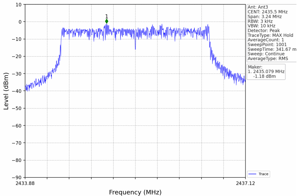
3M_MCH_2435.5MHz_Ant3_NTNV
