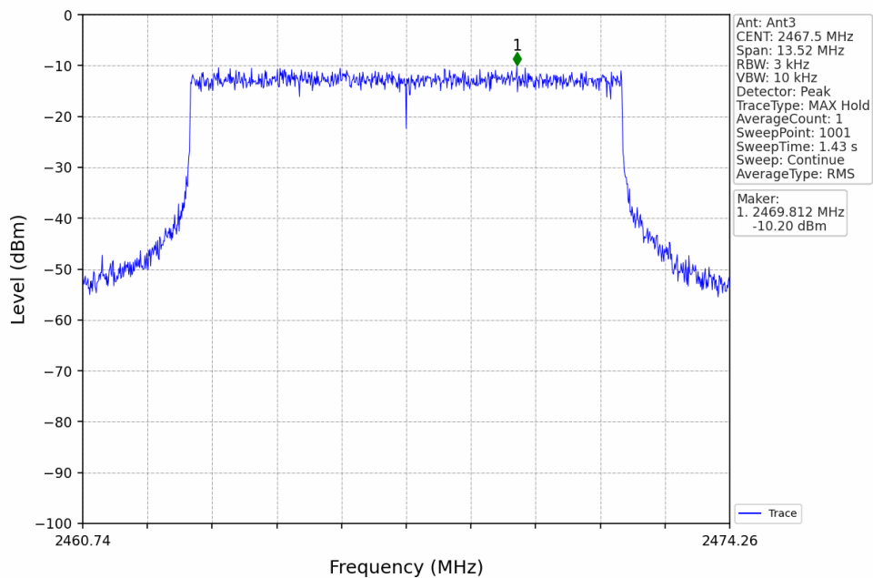
10M_HCH_2467.5MHz_Ant3_NTNV
