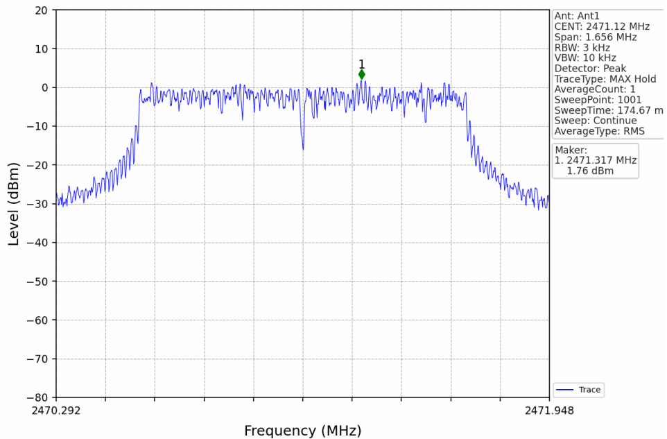
1.4M_HCH_2471.12MHz_Ant1_NTNV
