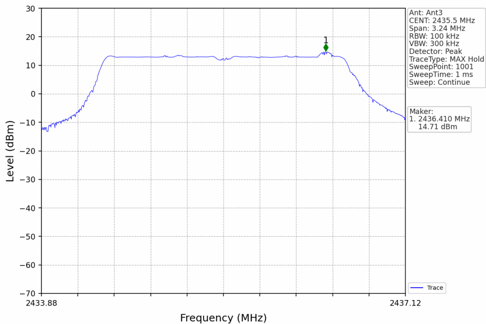
3M_MCH_2435.5MHz_Ant3_NTNV
