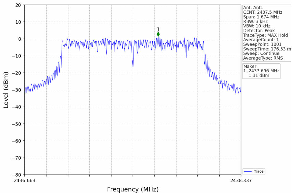
1.4M_MCH_2437.5MHz_Ant1_NTNV
