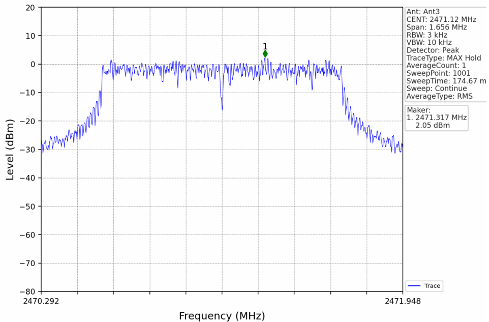
1.4M_HCH_2471.12MHz_Ant3_NTNV
