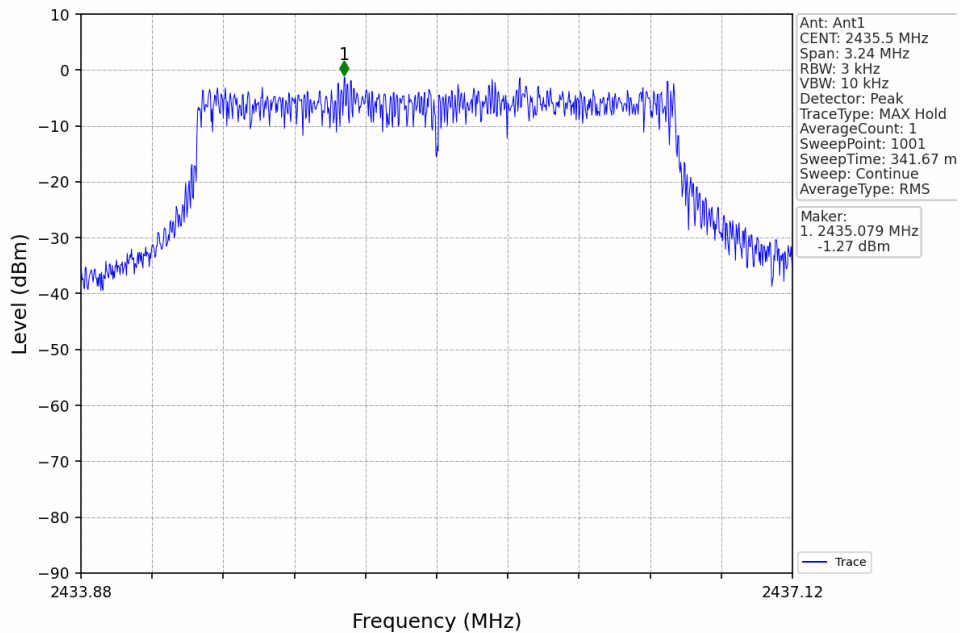
3M_MCH_2435.5MHz_Ant1_NTNV
