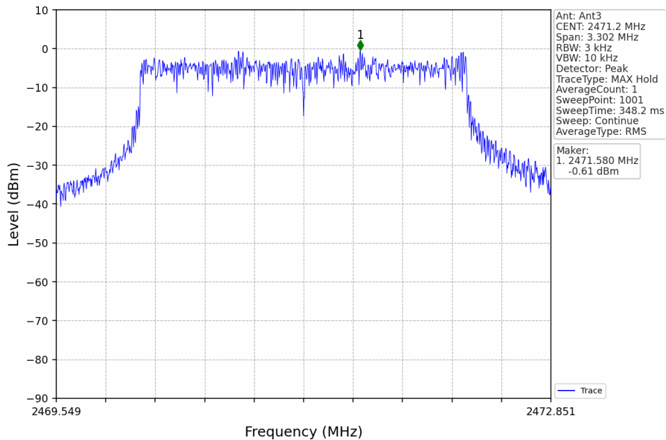
3M_HCH_2471.2MHz_Ant3_NTNV
