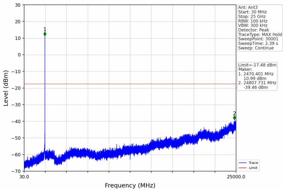
3M_HCH_2471.2MHz_Ant3_NTNV
