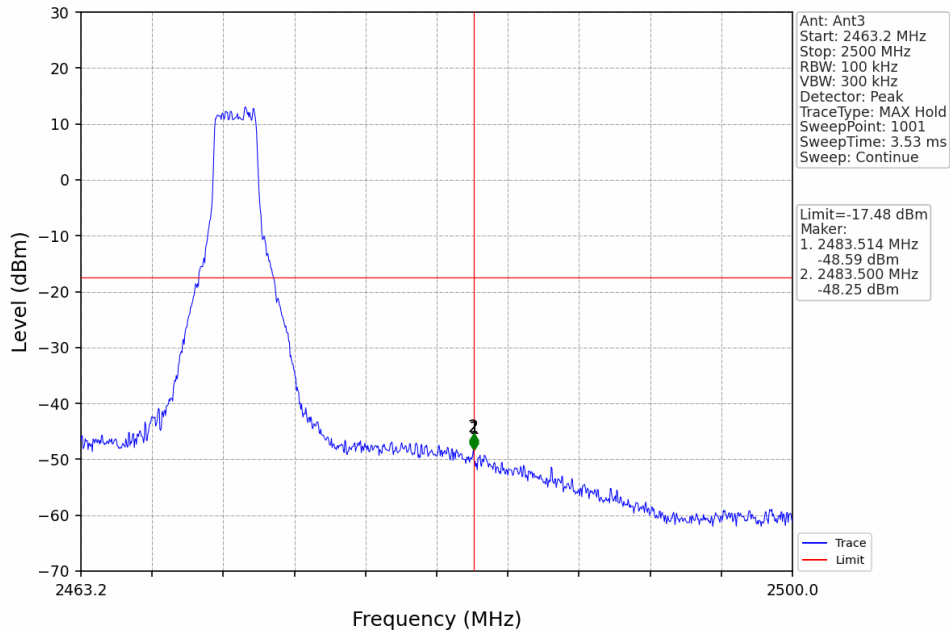
3M_HCH_2471.2MHz_Ant3_NTNV
