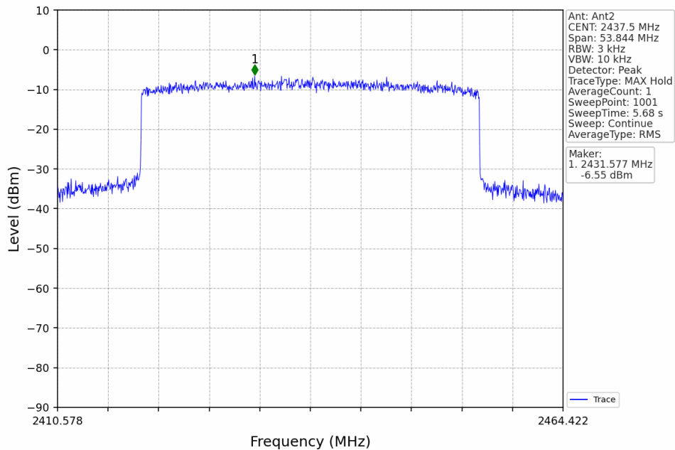
40M_MCH_2437.5MHz_Ant2_NTNV
