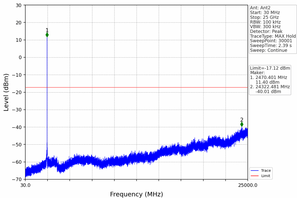
3M_HCH_2471.2MHz_Ant2_NTNV
