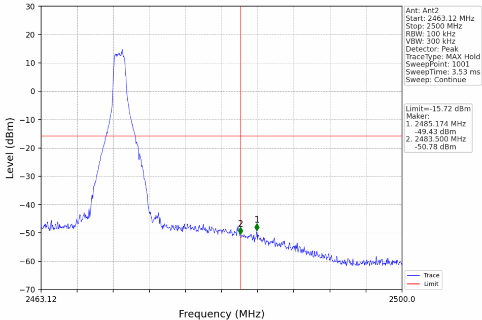
1.4M_HCH_2471.12MHz_Ant2_NTNV
