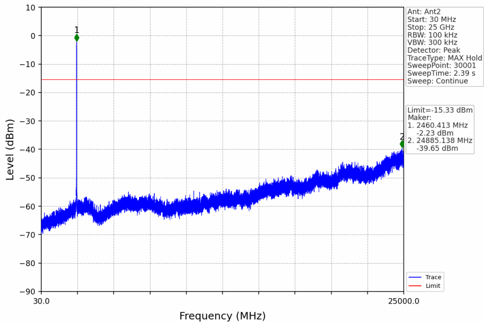
20M_HCH_2462.5MHz_Ant2_NTNV
