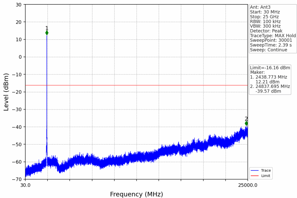
10M_MCH_2437.5MHz_Ant3_NTNV
