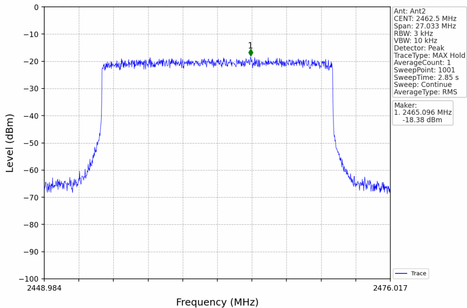
20M_HCH_2462.5MHz_Ant2_NTNV
