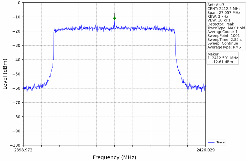
20M_LCH_2412.5MHz_MIMO_NTNV
