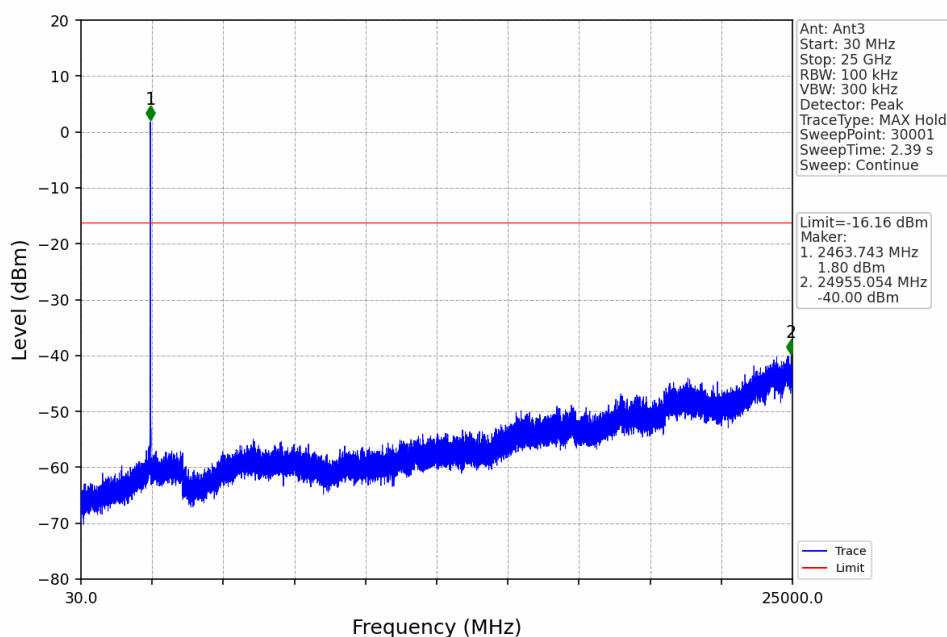
10M_HCH_2467.5MHz_Ant3_NTNV
