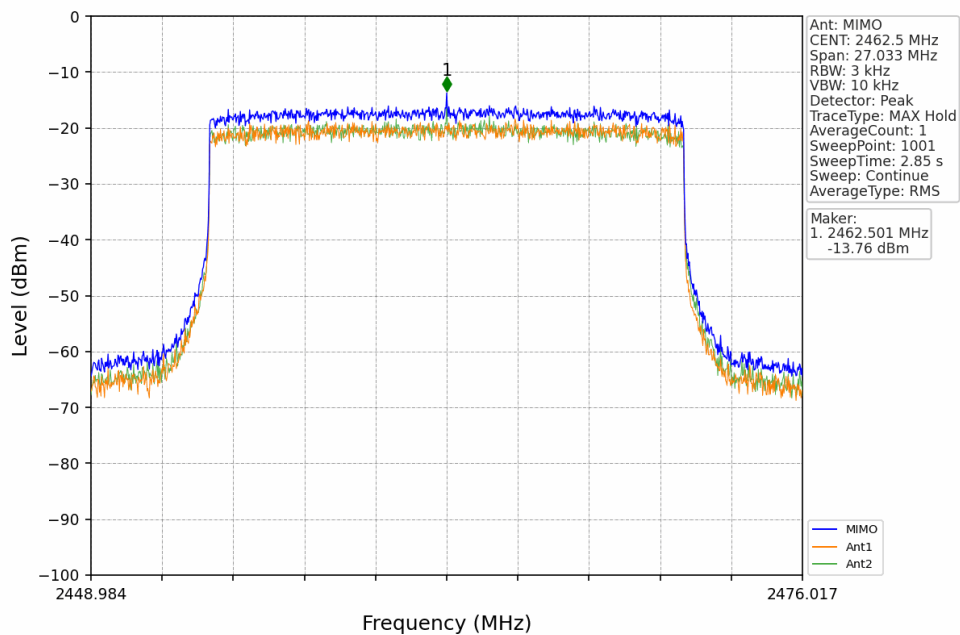
20M_HCH_2462.5MHz_MIMO_NTNV
