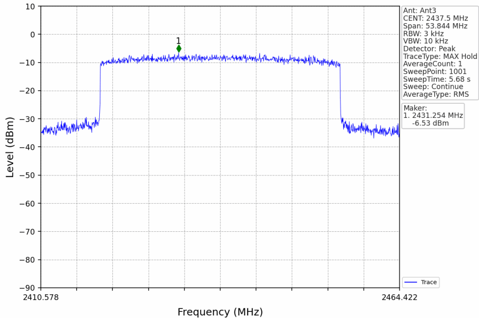
40M_MCH_2437.5MHz_MIMO_NTNV
