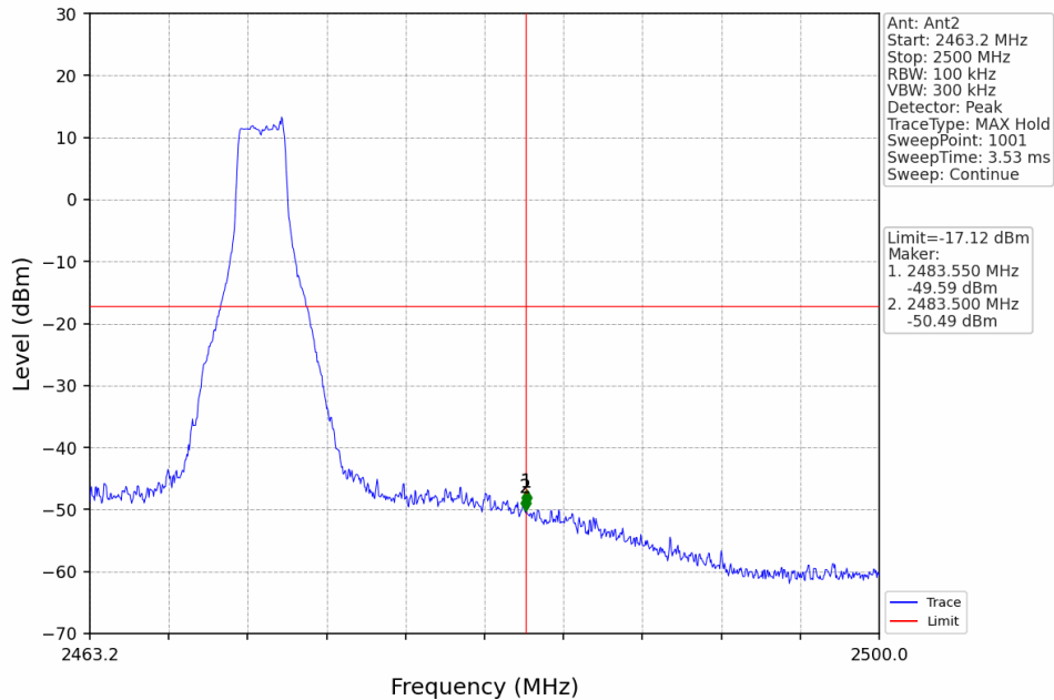
3M_HCH_2471.2MHz_Ant2_NTNV
