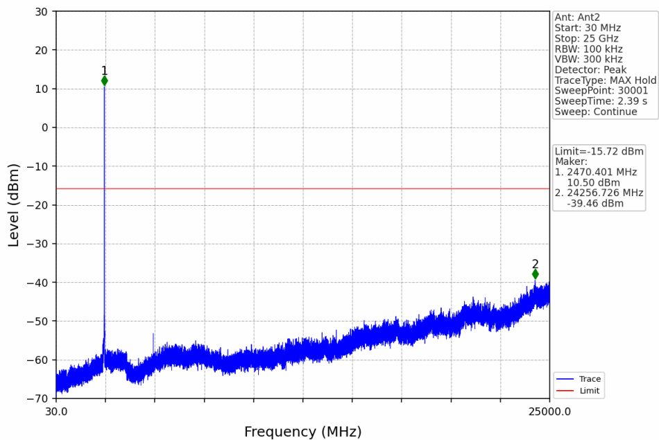
1.4M_HCH_2471.12MHz_Ant2_NTNV
