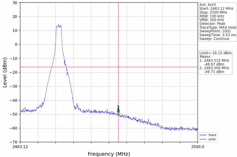
1.4M_HCH_2471.12MHz_Ant3_NTNV
