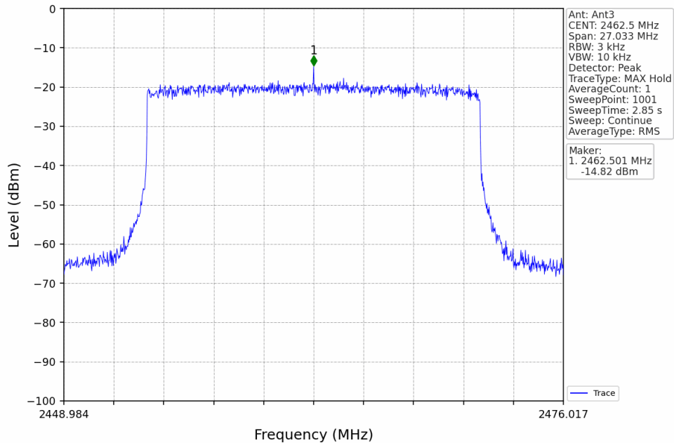
20M_HCH_2462.5MHz_MIMO_NTNV
