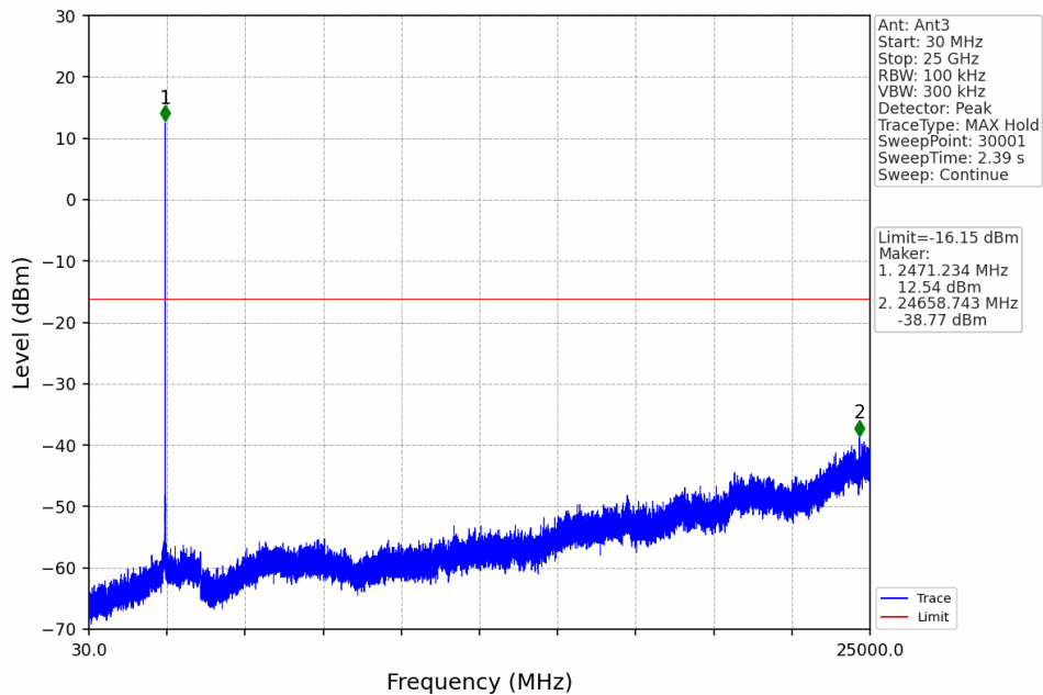
1.4M_HCH_2471.12MHz_Ant3_NTNV
