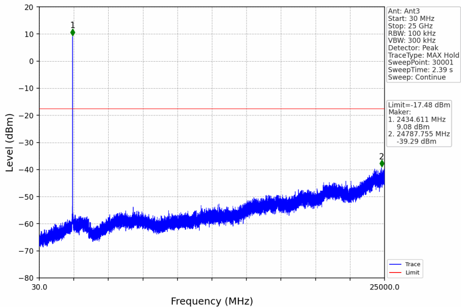
3M_MCH_2435.5MHz_Ant3_NTNV
