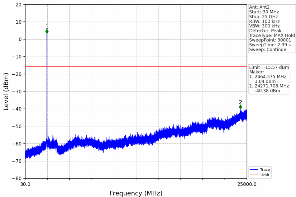
10M_HCH_2467.5MHz_Ant2_NTNV
