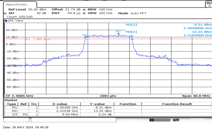
SRD 10M Ant1 2408.5
