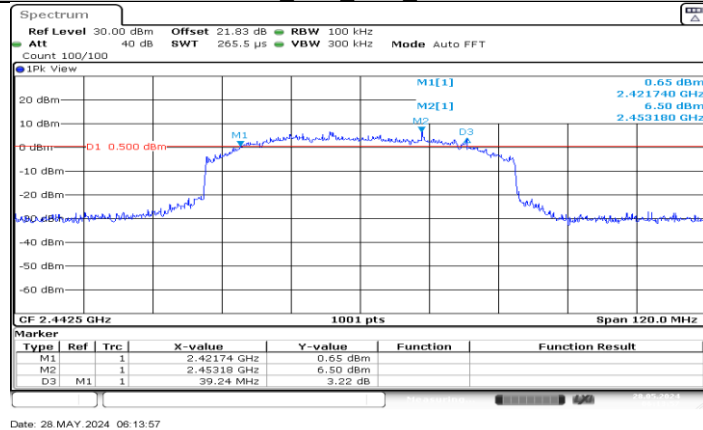
SRD 60M Ant1 2442.5
