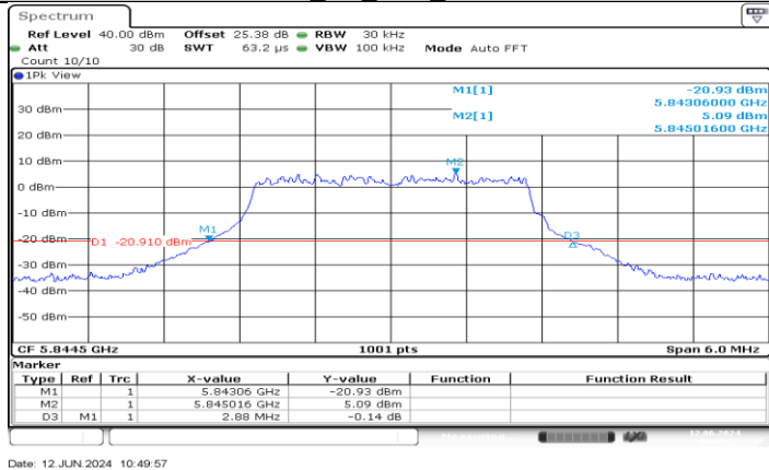
SRD_3M_Ant2_5844.5
