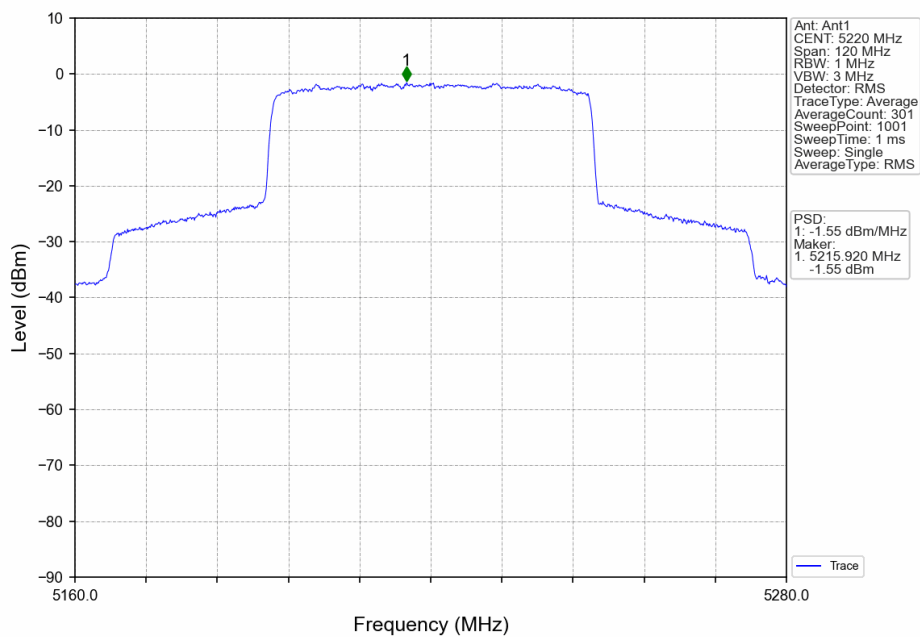
60M_HCH_5220MHz_Ant1_NTNV
