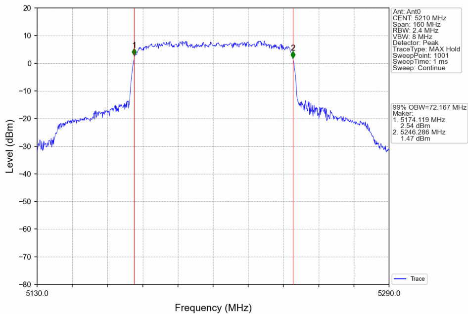
80M_HCH_5210MHz_Ant0_NTNV
