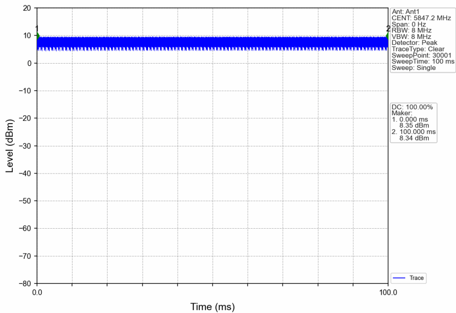
3M_HCH_5847.2MHz_Ant1_NTNV
