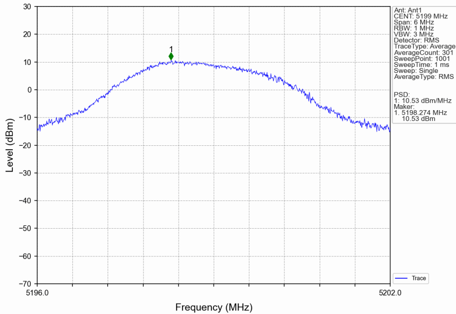
3M_MCH_5199MHz_Ant1_NTNV
