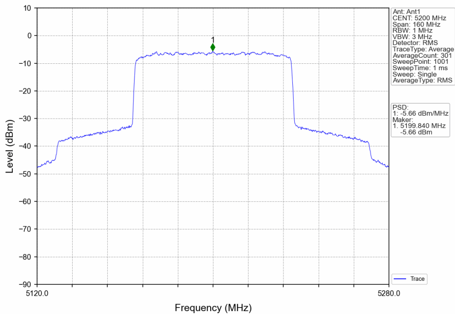
80M_MCH_5200MHz_Ant1_NTNV
