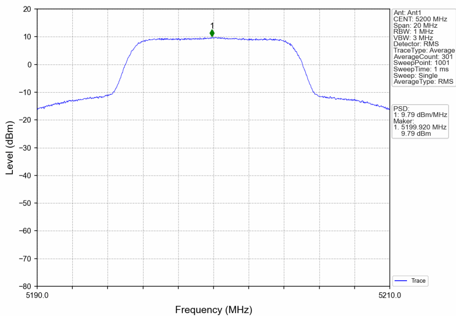
10M_MCH_5200MHz_Ant1_NTNV
