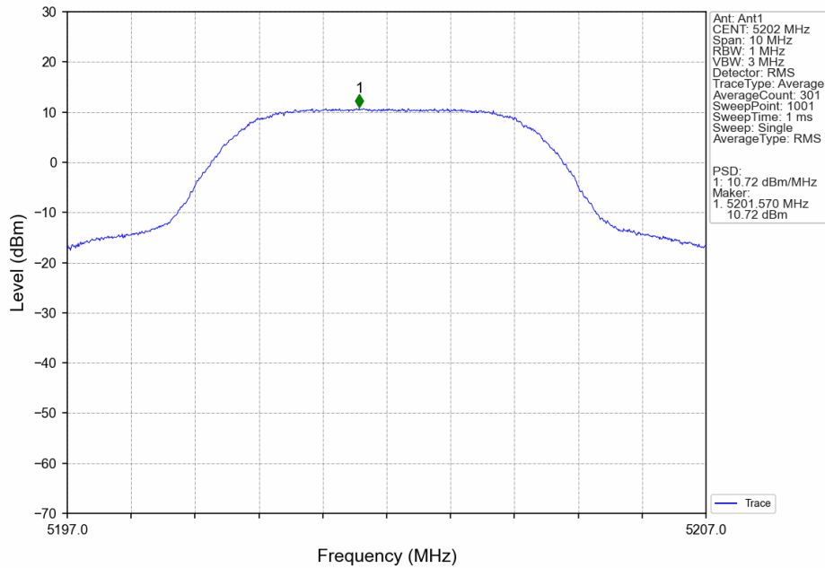
5M_MCH_5202MHz_Ant1_NTNV
