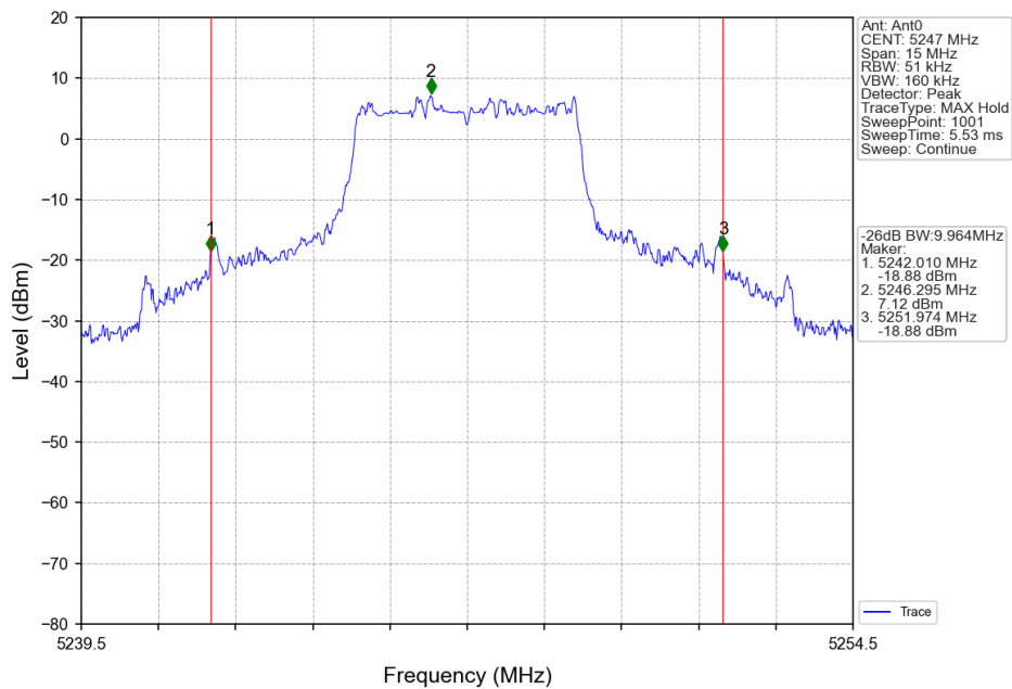
5M_HCH_5247MHz_Ant0_NTNV
