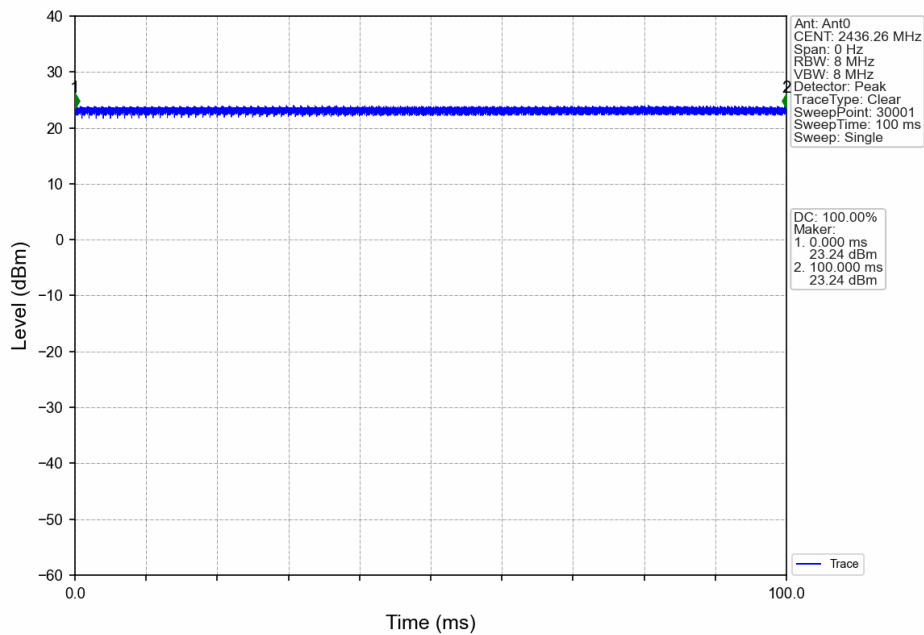
5M_MCH_2436.26MHz_Ant0_NTNV
