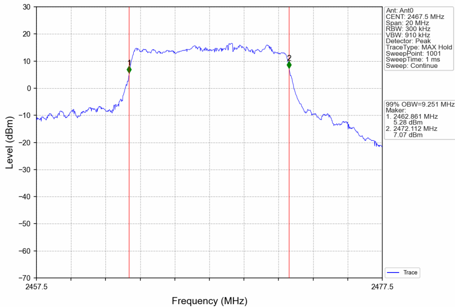
10M_HCH_2467.5MHz_Ant0_NTNV
