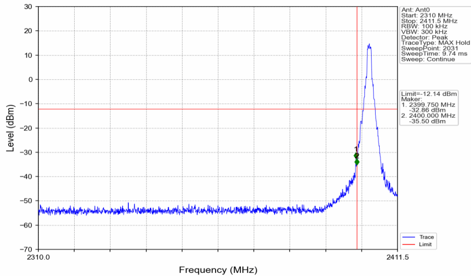
1.4M_LCH_2403.5MHz_Ant0_NTNV
