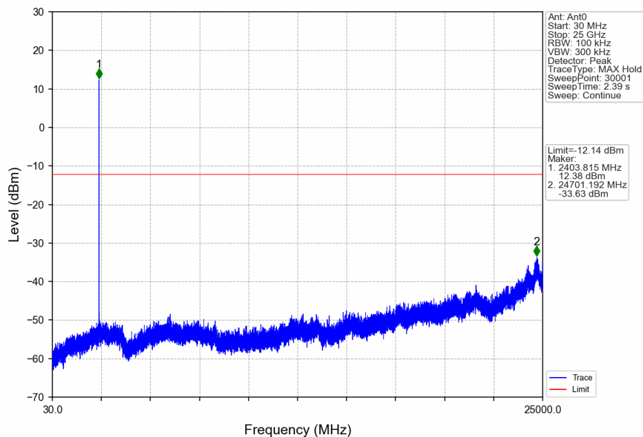
1.4M_LCH_2403.5MHz_Ant0_NTNV
