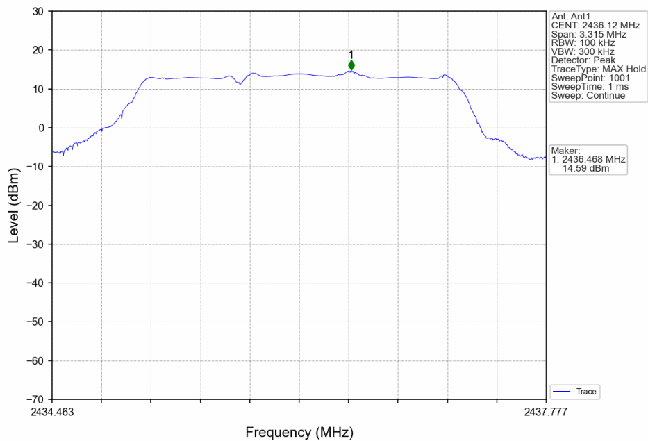
3M_MCH_2436.12MHz_Ant1_NTNV
