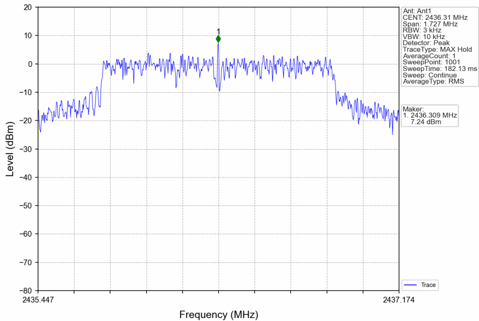
1.4M_MCH_2436.31MHz_Ant1_NTNV
