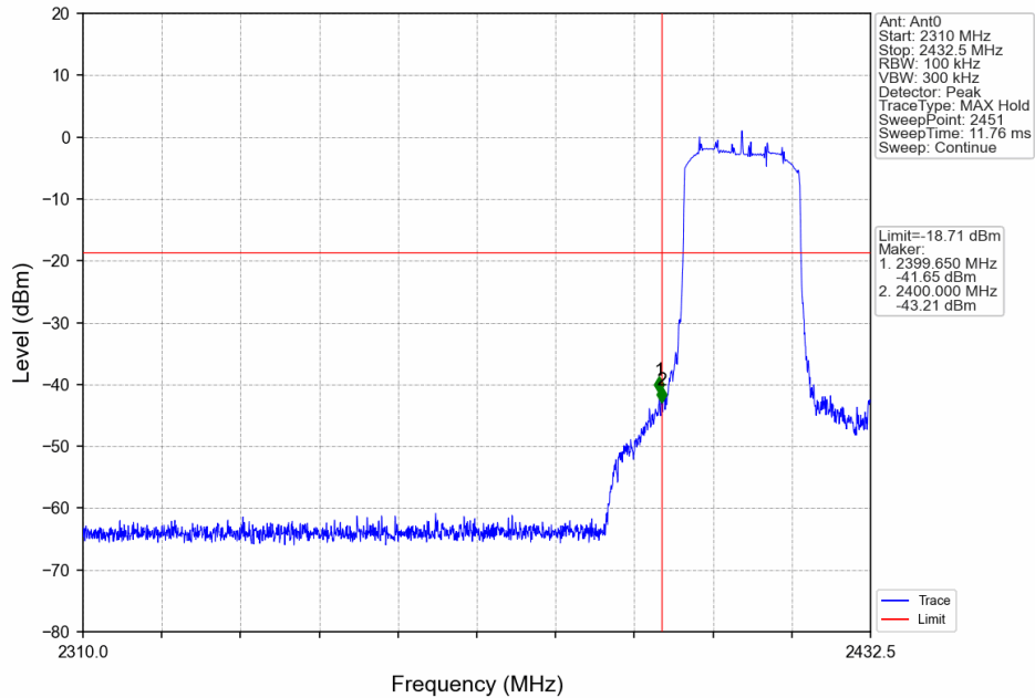
20M_LCH_2412.5MHz_Ant0_NTNV
