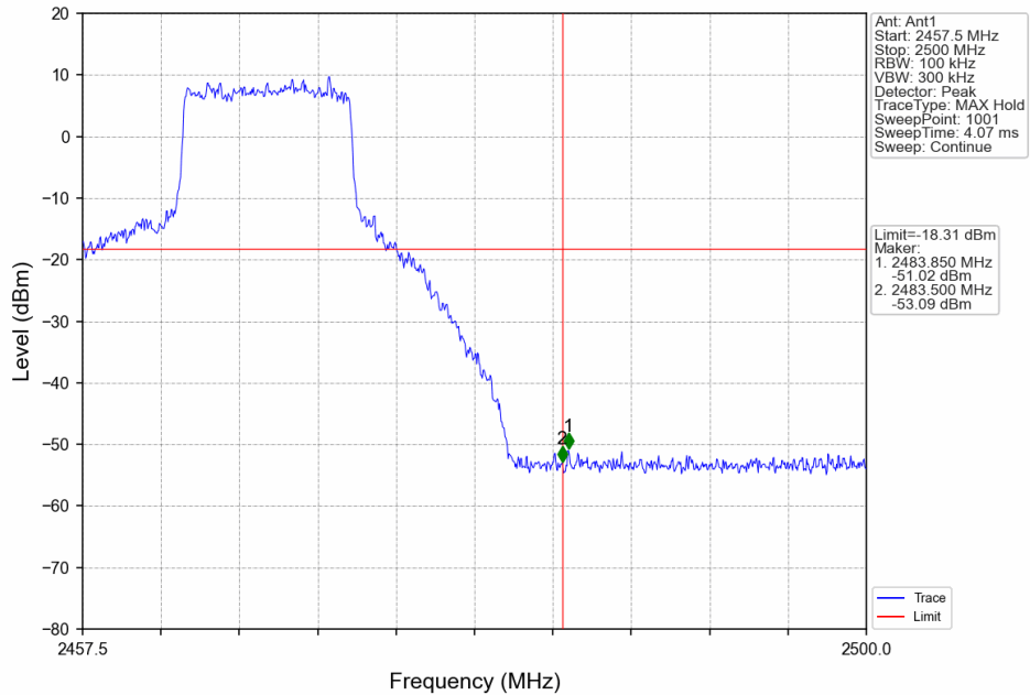
10M_HCH_2467.5MHz_Ant1_NTNV
