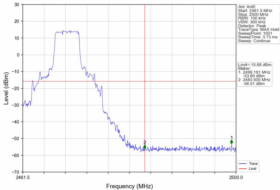
5M_HCH_2469.5MHz_Ant0_NTNV
