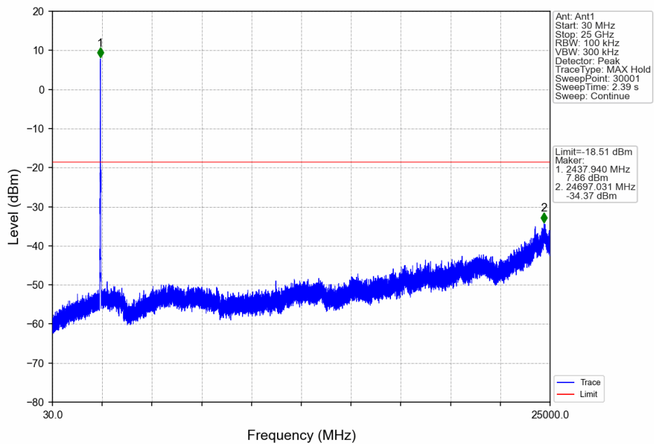
20M_MCH_2437.5MHz_Ant1_NTNV
