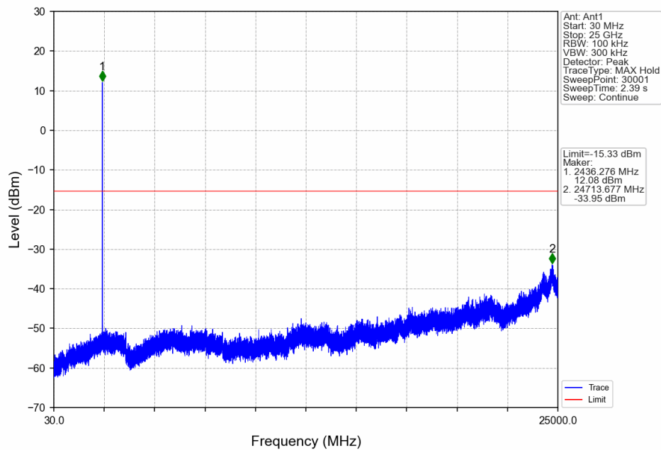
5M_MCH_2436.26MHz_Ant1_NTNV
