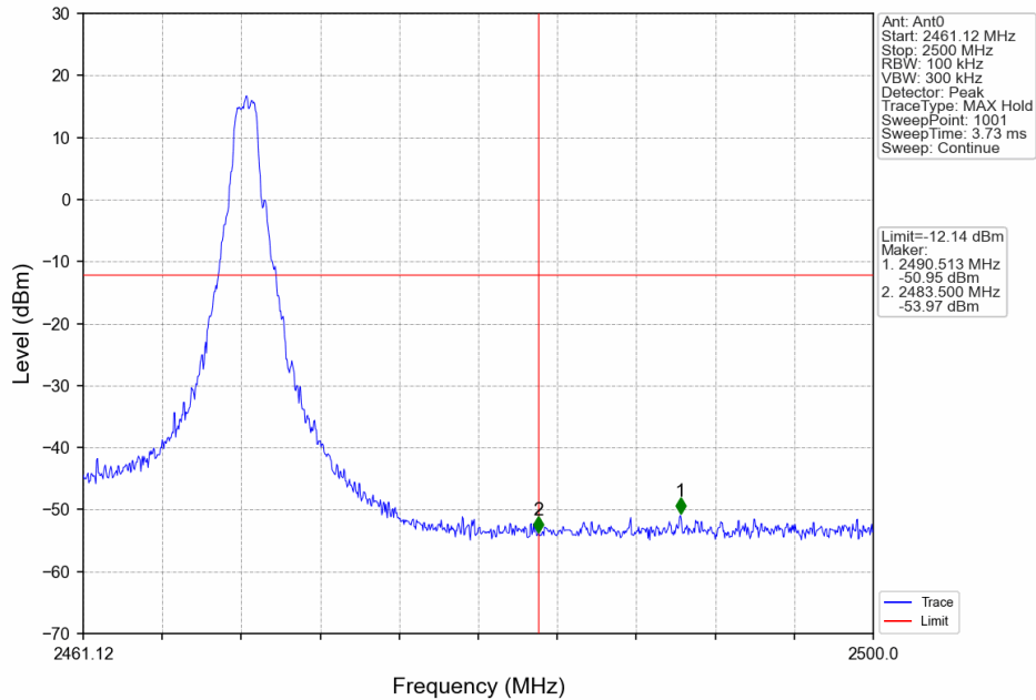
1.4M_HCH_2469.12MHz_Ant0_NTNV
