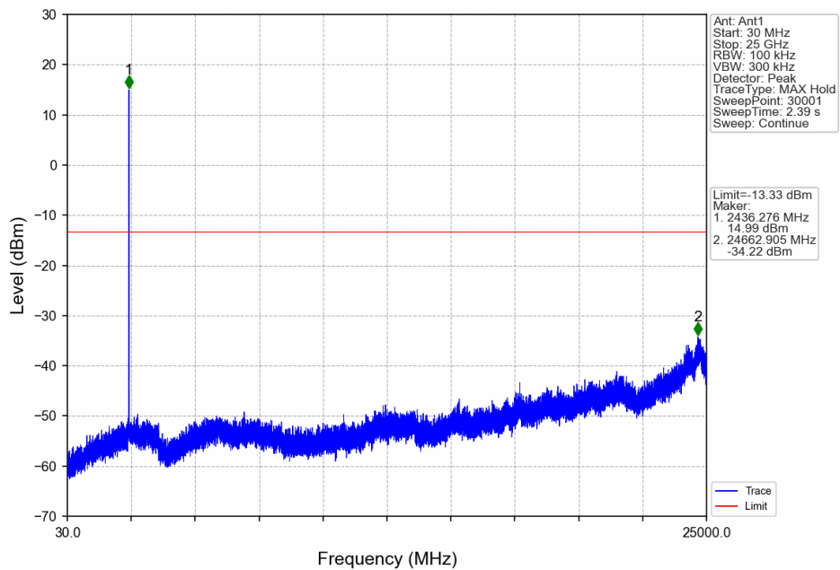
3M_MCH_2436.12MHz_Ant1_NTNV
