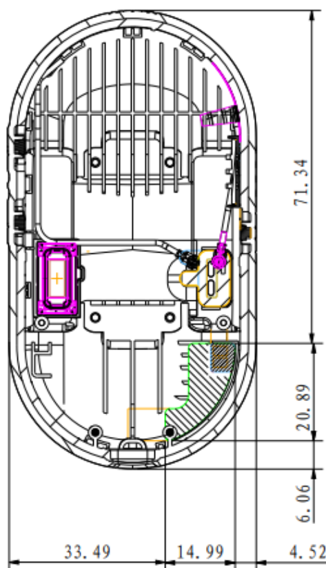
BLE/Wi-Fi Antenna
