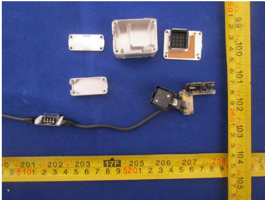
EUT – IMU PRO Module Uncover View
