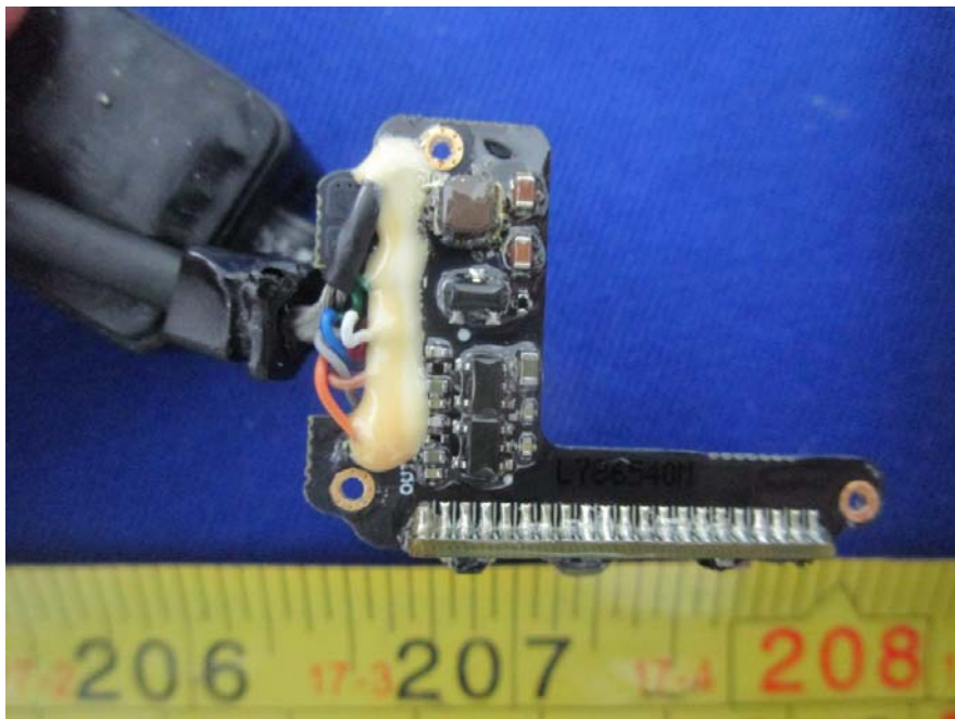
EUT – IMU PRO Module Sub-board Bottom View
