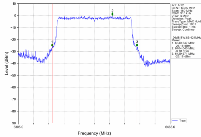
802.11ax(HEW80) HCH_6385MHz_SU / Ant2 NTN
