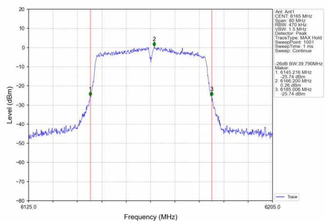
802.11ac(VHT40) MCH_6165MHz_Ant1_NTNV
