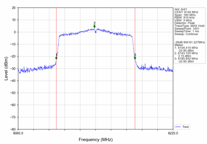
802.11ac(VHT80) MCH_6145MHz_Ant1_NTNV
