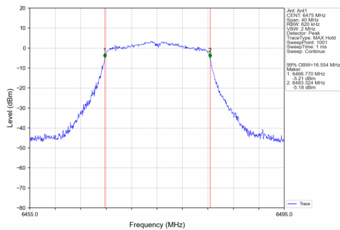
802.11a_MCH_6475MHz_Ant1_NTNV
