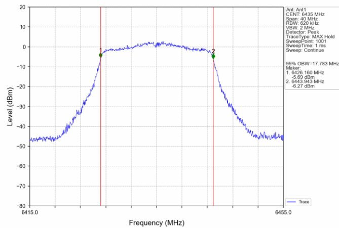
802.11ac(VHT20)_LCH_6435MHz_Ant1_NTNV
