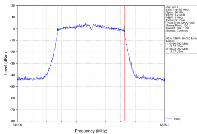
802.11n(HT40) MCH 6485MHz Ant1 NTN
