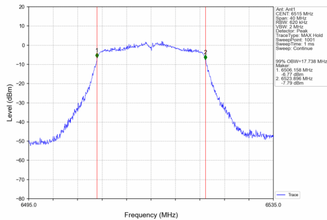
802.11n(HT20) HCH_6515MHz_Ant1_NTNV
