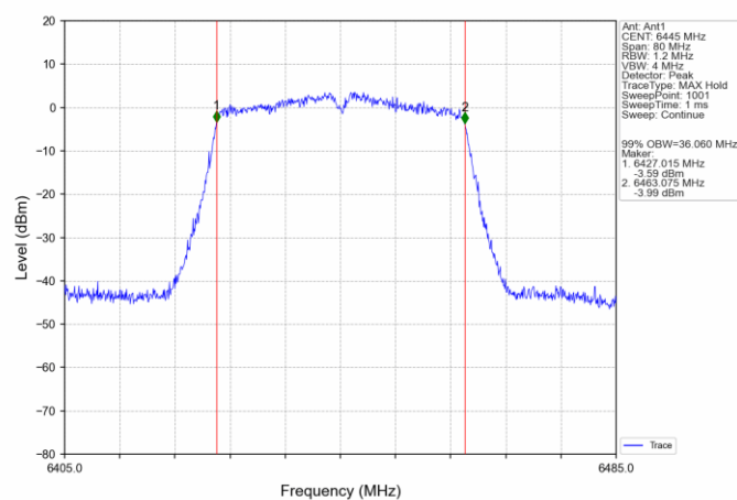
802.11ac(VHT40) LCH 6445MHz Ant1_NTNV
