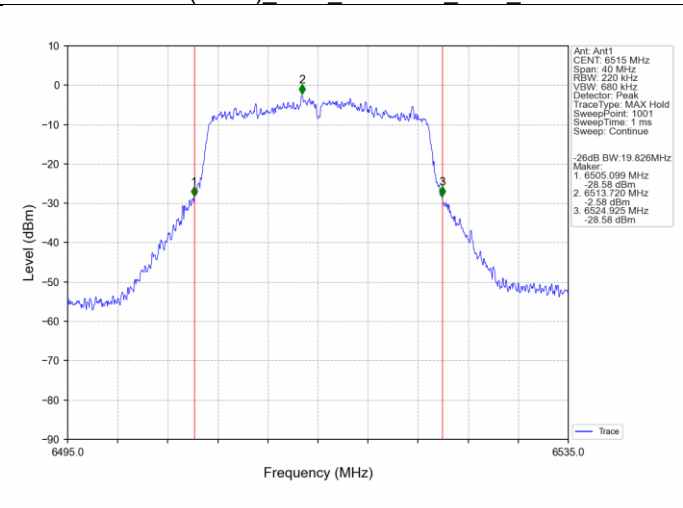
802.11n(HT20) HCH_6515MHz_Ant1_NTNV
