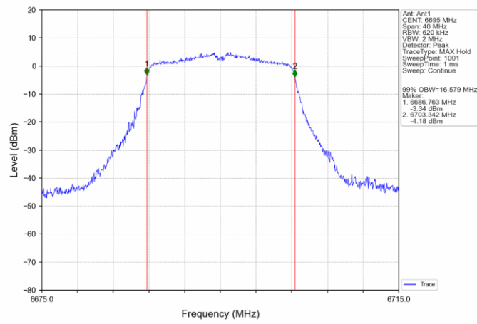
802.11a MCH_6695MHz_Ant1_NTNV
