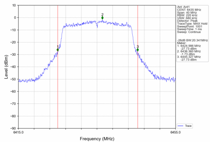
802.11ac(VHT20)_LCH_6435MHz_Ant1_NTNV
