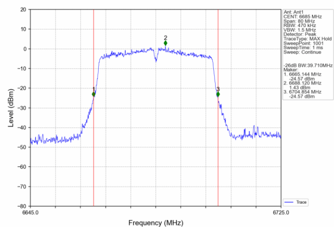
802.11ac(VHT40) MCH_6685MHz_Ant1_NTNV
