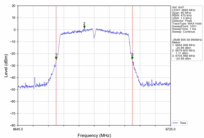
802.11n(HT40) MCH_6685MHz_Ant1_NTNV
