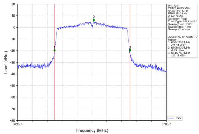
802.11ac(VHT80)_MCH_6705MHz_Ant1_NTNV
