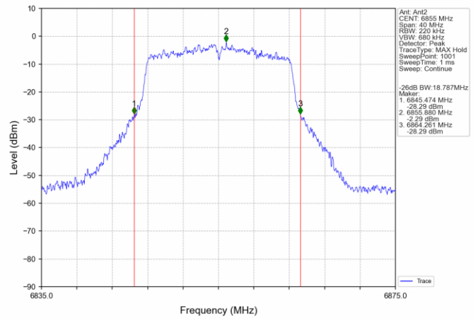
802.11a_HCH_6855MHz_Ant2_NTNV
