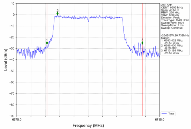
802.11ax(HEW20) MCH 6695MHz SU / Ant1 NTN
