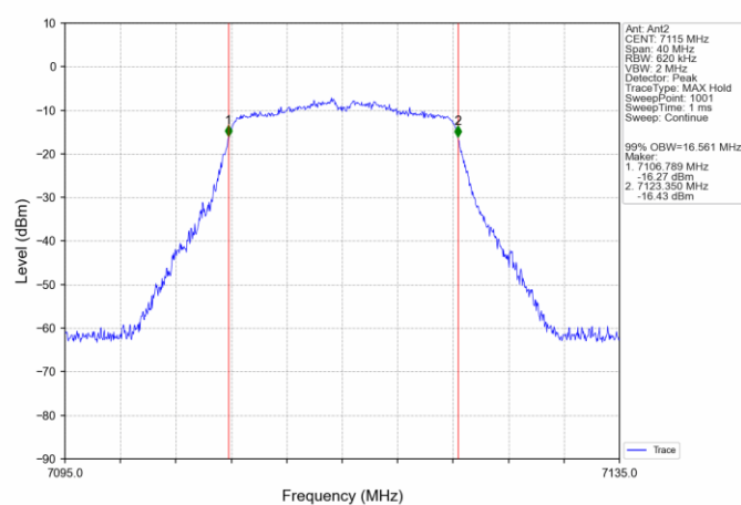
802.11a_HCH_7115MHz_Ant2_NTNV
