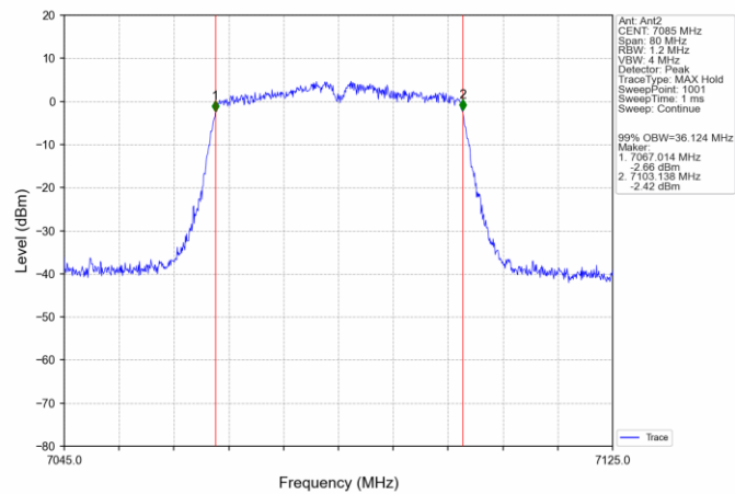
802.11ac(VHT40) HCH_7085MHz_Ant2_NTNV
