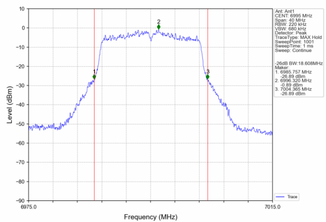
802.11a_MCH_6995MHz_Ant1_NTNV
