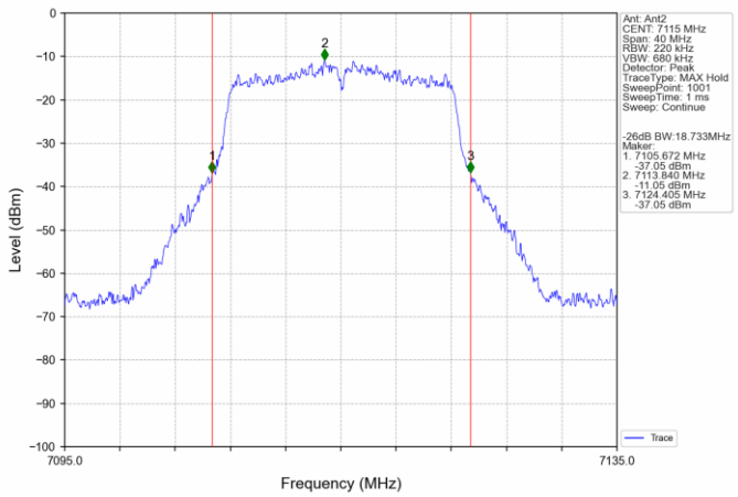
802.11a_HCH_7115MHz_Ant2_NTNV
