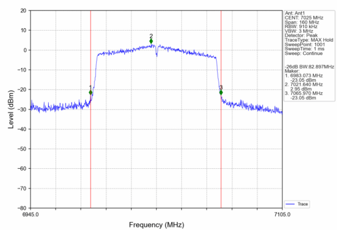
802.11ac(VHT80) HCH_7025MHz_Ant1_NTNV
