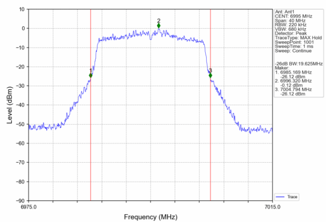
802.11n(HT20)_MCH_6995MHz_Ant1_NTNV
