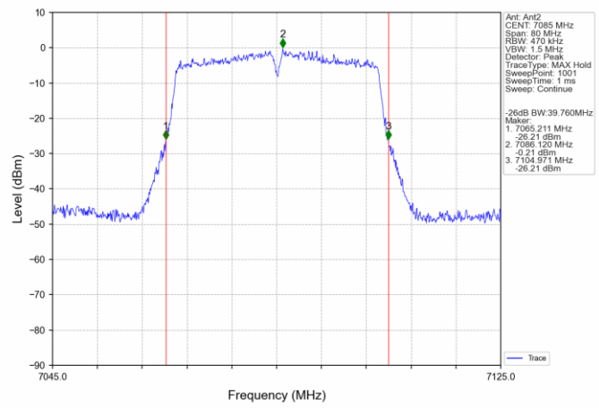
802.11ac(VHT40) HCH_7085MHz_Ant2_NTNV
