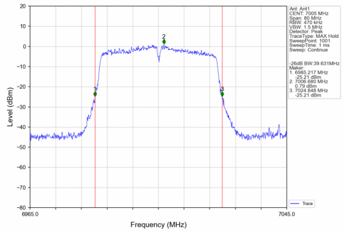
802.11ac(VHT40) MCH_7005MHz_Ant1_NTNV
