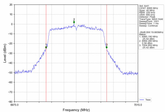
802.11ac(VHT20) MCH 6995MHz Ant1 NTN
