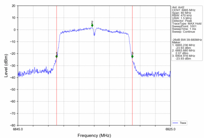
802.11n(HT40) HCH 6885MHz Ant2 NTN
