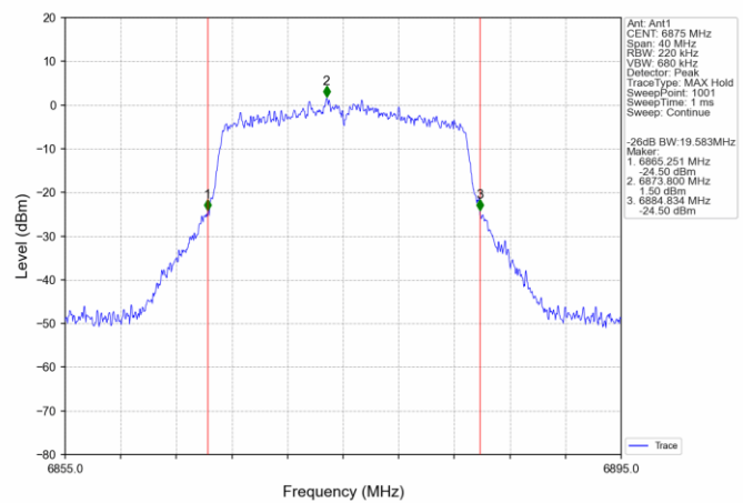
802.11n(HT20)_HCH_6875MHz_Ant1_NTNV
