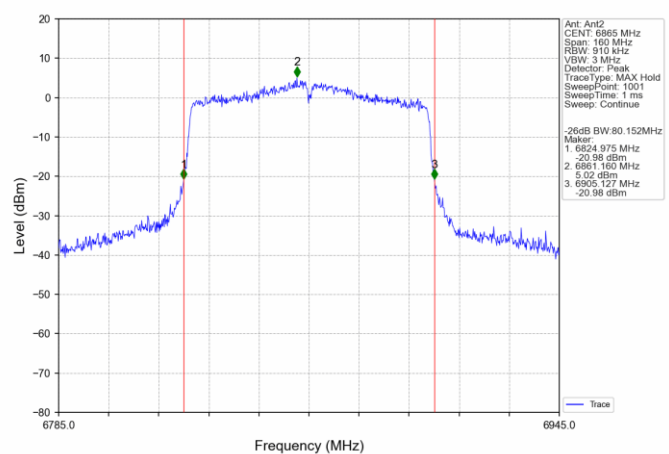
802.11ac(VHT80) HCH_6865MHz_Ant2_NTNV
