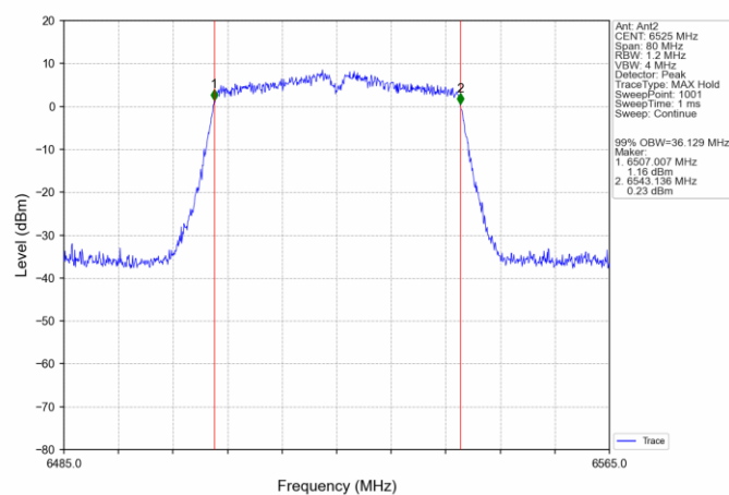
802.11ac(VHT40) HCH_6525MHz_Ant2_NTNV
