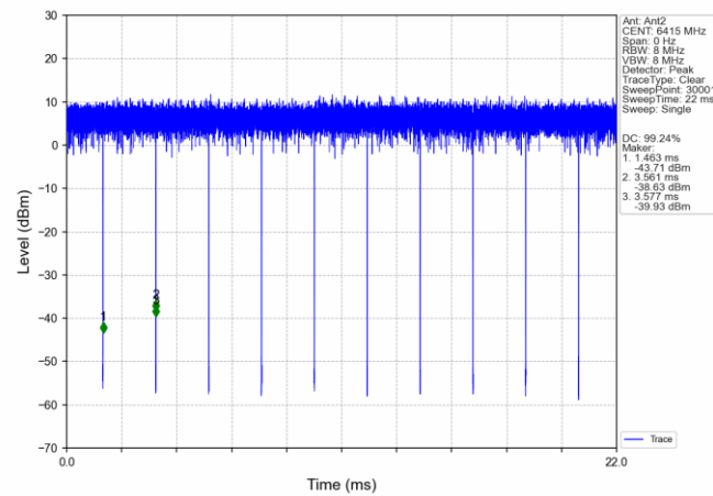
802.11a_HCH_6415MHz_Ant2_NTNV
