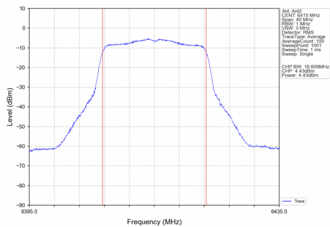
802.11a_HCH_6415MHz_Ant2_NTNV
