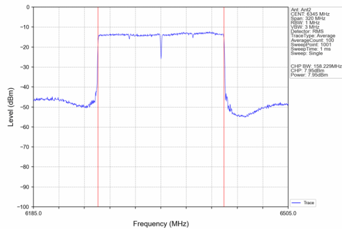
802.11ax(HEW160) HCH 6345MHz SU / Ant2 NTN
