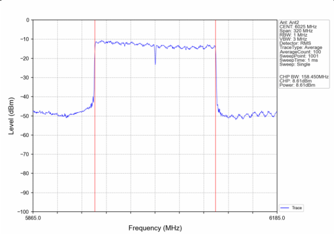
802.11ax(HEW160) LCH 6025MHz SU / Ant2 NTN
