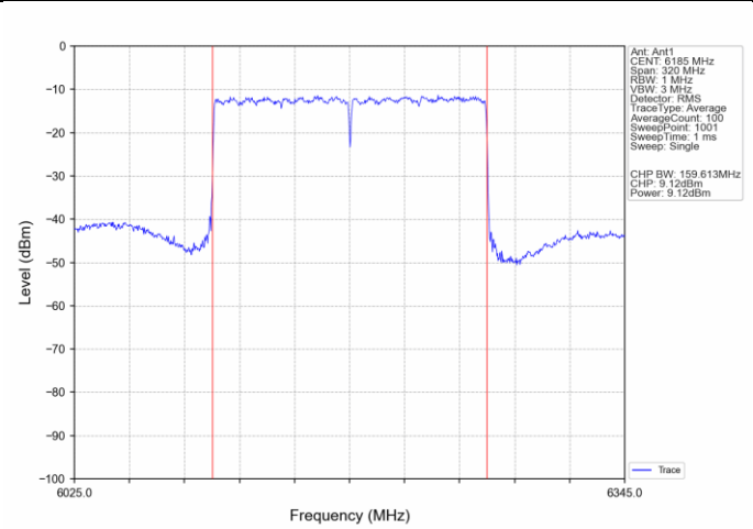
802.11ax(HEW160) MCH 6185MHz SU / Ant1 NTN
