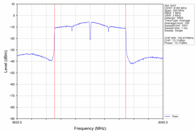
802.11ac(VHT160) MCH 6185MHz Ant1 NTN
