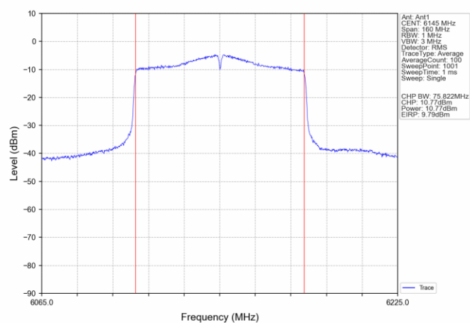
802.11ac(VHT80) MCH_6145MHz_Ant1_NTNV
