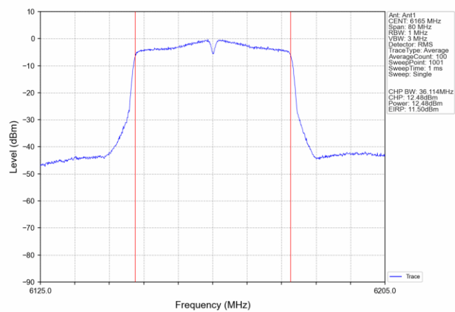
802.11n(HT40) MCH_6165MHz_Ant1_NTNV
