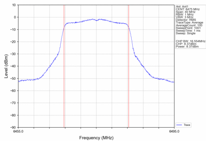
802.11a_MCH_6475MHz_Ant1_NTNV
