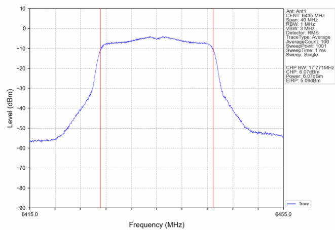
802.11ac(VHT20) LCH_6435MHz_Ant1_NTNV
