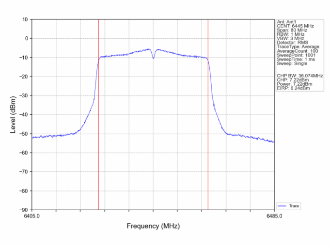
802.11ac(VHT40) LCH 6445MHz Ant1_NTNV
