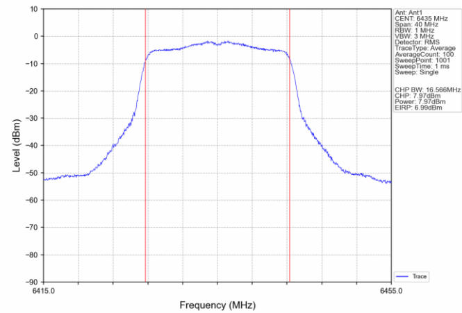
802.11a LCH 6435MHz Ant1 NTN
