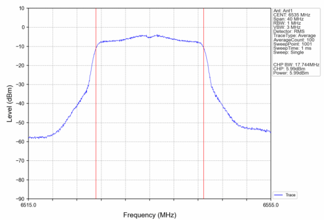
802.11ac(VHT20) LCH_6535MHz_Ant1_NTNV
