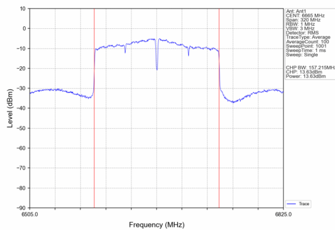
802.11ac(VHT160) MCH_6665MHz_Ant1_NTNV
