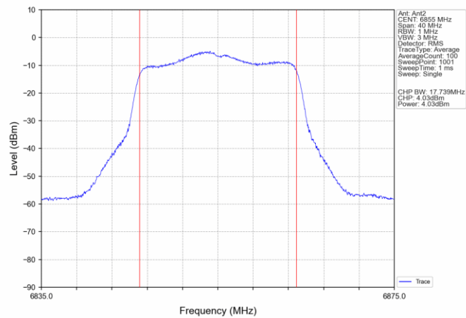
802.11n(HT20) HCH 6855MHz Ant2 NTN
