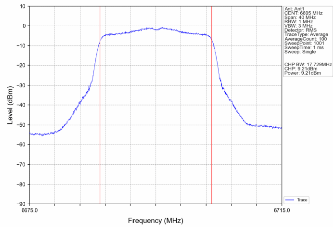
802.11ac(VHT20) MCH_6695MHz_Ant1_NTNV
