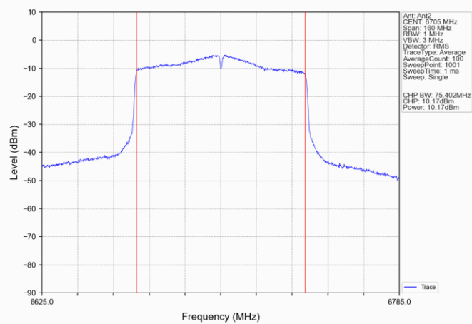
802.11ac(VHT80) MCH 6705MHz Ant2 NTN
