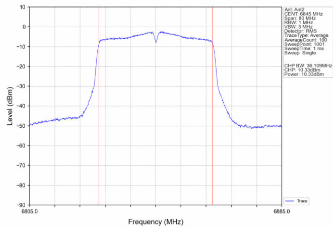
802.11n(HT40) HCH 6845MHz_Ant2_NTNV
