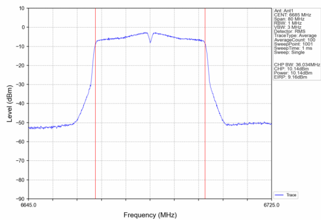
802.11n(HT40) MCH_6685MHz_Ant1_NTNV
