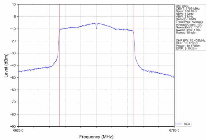
802.11ac(VHT80) MCH 6705MHz Ant2 NTN
