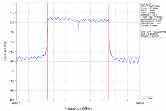
802.11ax(HEW160) MCH 6665MHz SU / Ant2 NTV
