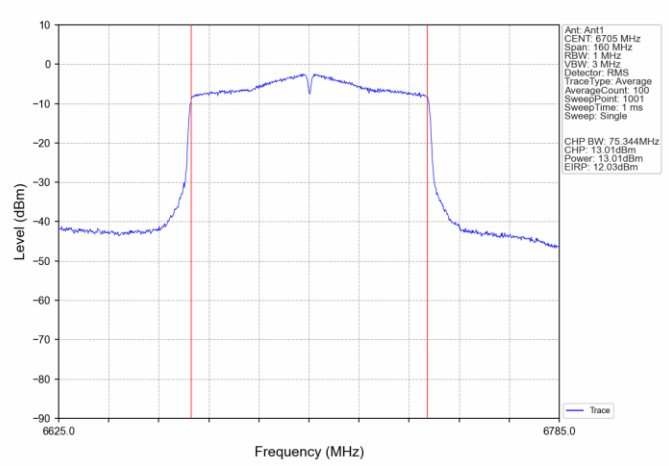
802.11ac(VHT80) MCH_6705MHz_Ant1_NTNV
