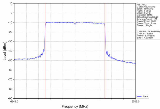
802.11ax(HEW80) LCH 6625MHz SU / Ant2 NTN
