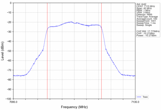
802.11n(HT20) HCH 7115MHz Ant2 NTN
